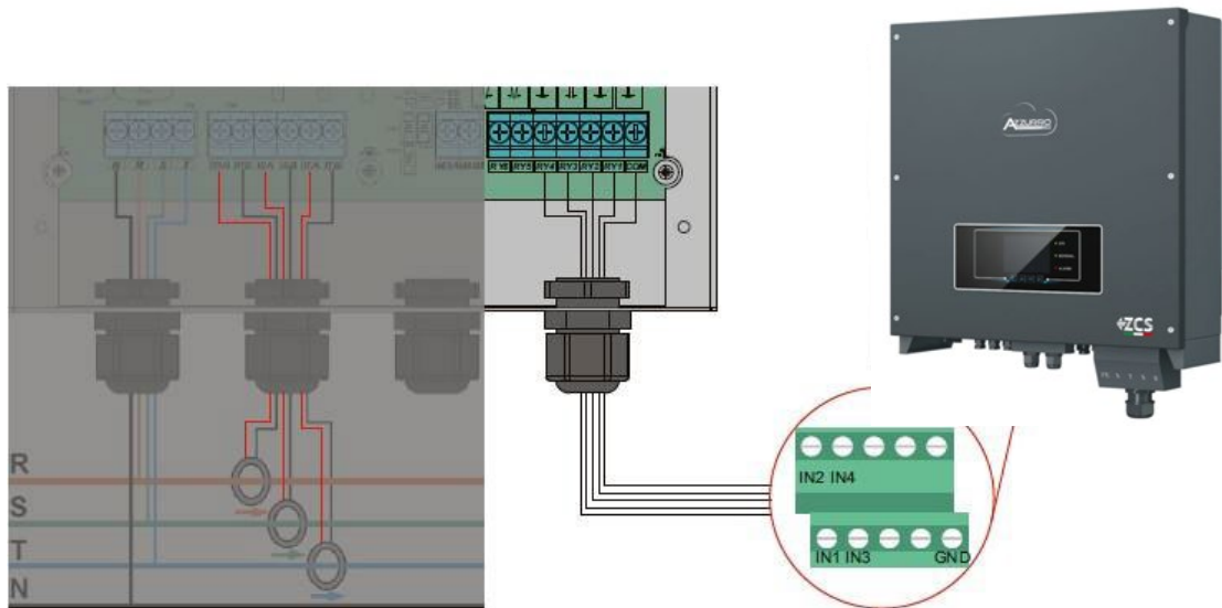
Figura 6 - Conexiones de comunicación dispositivo ARPC
