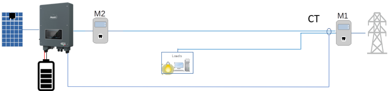
Abbildung 3 - Logische Position des Stromsensors im Fall von 2 Phasen, die vom Zähler M1 abgehen
