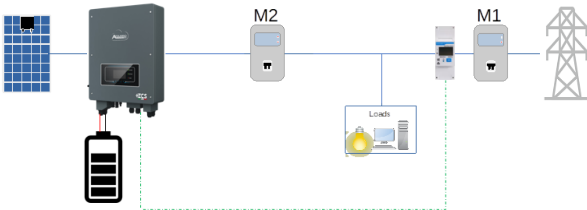
Abbildung 1 - Logische Position des Messgeräts DDSU666
