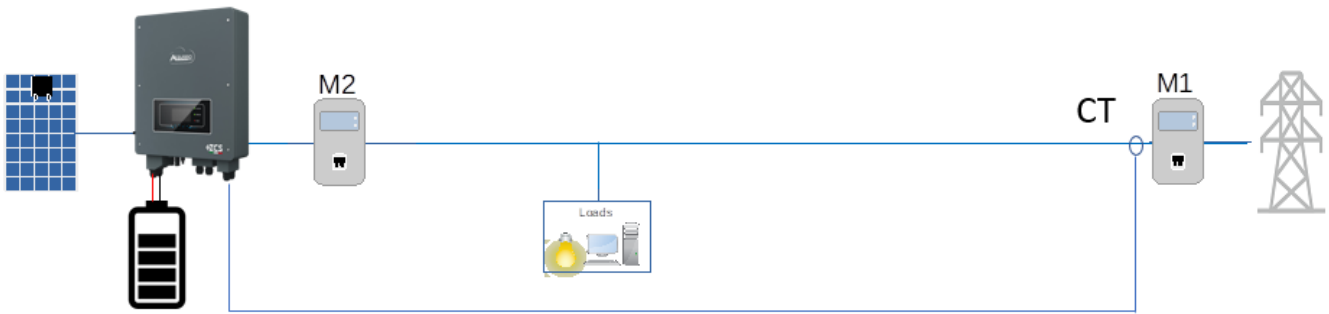
Abbildung 2 - Logische Position des Stromsensors im Fall einer einzigen Phase, die vom Zähler M1 abgeht
