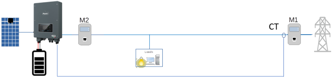
Рисунок 2 - логічне положення ТА у разі відключення однієї фази від лічильника M1
