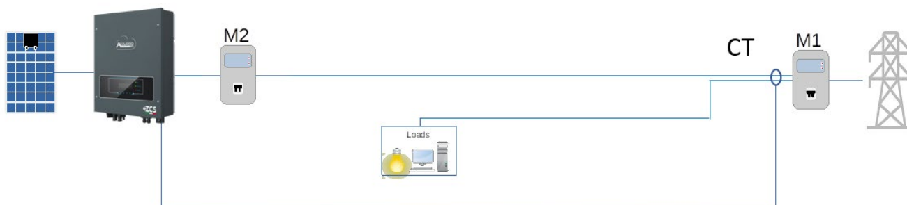
Figura 3 - posición lógica del TA en caso de que del contador M1 salgan 2 fases.
