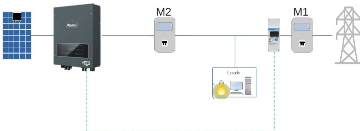
Figura 1 - posición lógica del medidor DDSU666
