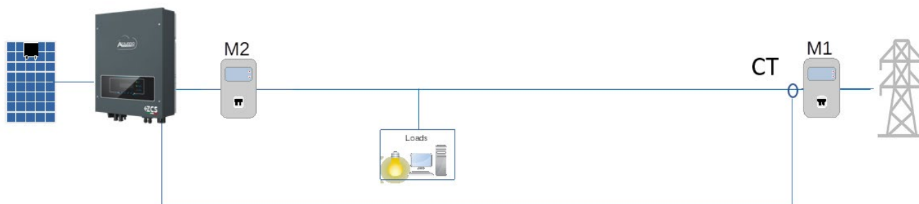
Figura 2 - posición lógica del TA en caso de que del contador M1 salga una única fase
