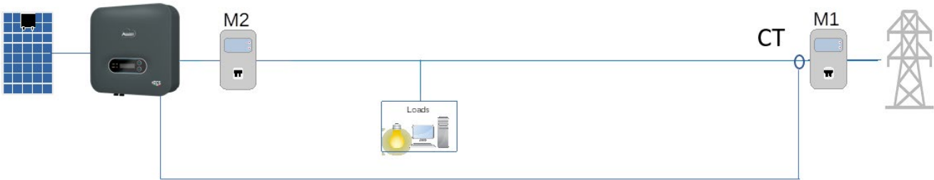
Рисунок 2 - логічне положення ТА у разі відключення однієї фази від лічильника M1
