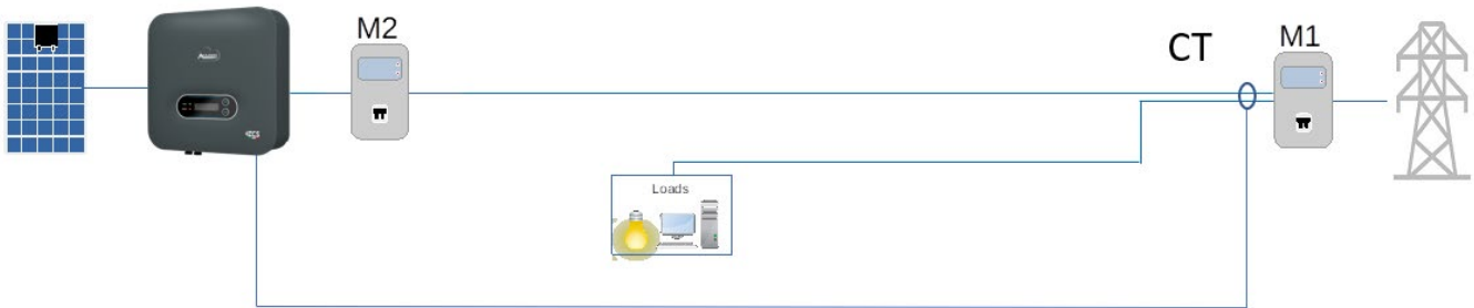
Рисунок 3 - логічне положення ТА у разі відключення двох фаз від лічильника M1
