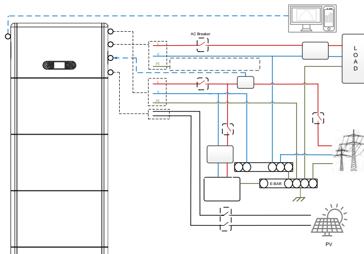
Figura 55 - Topologia elettrica del sistema (versione australiana)
