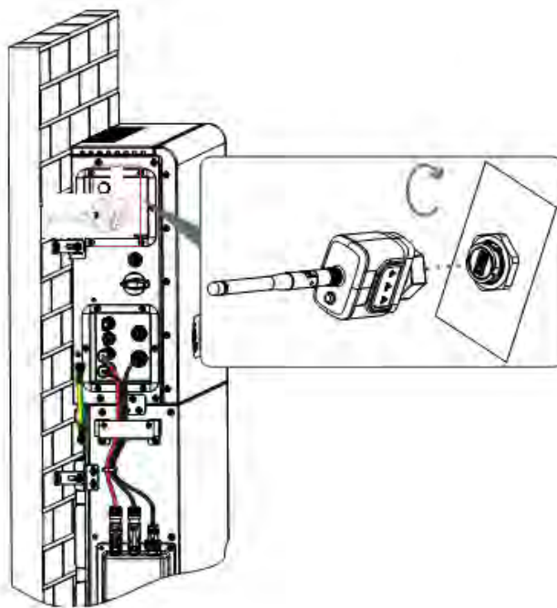
Figura 25 - Collegamento WIFI/4G
