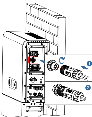
Figura 31 - Collegamento EPS
