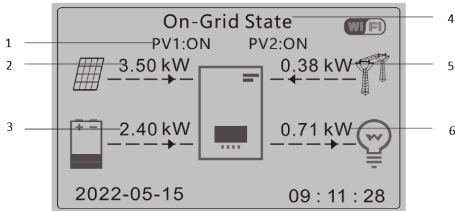
Figura 59 - Interfaccia principale
