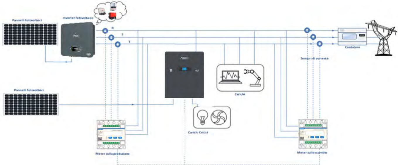
Figura 48 - Schema di installazione ibrida con Meter DTSU trifase in scambio e produzione
