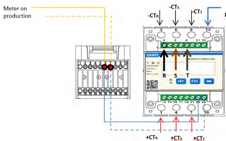
Figura 49 - Connessione della porta seriale COM con più di un Meter DTSU
