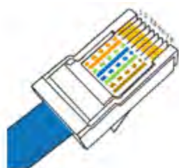
Figura 100 – Pin in uscita per il collegamento del connettore RJ45
