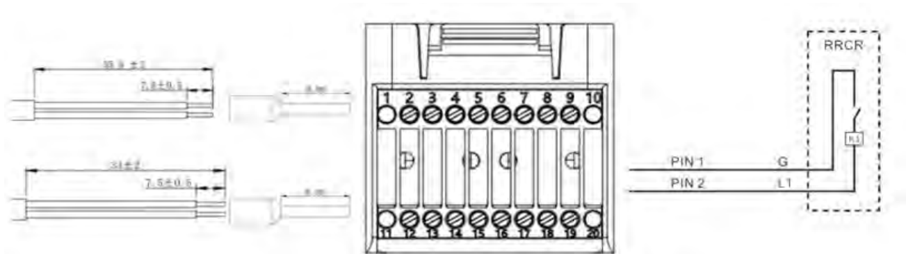
Figura 41 - Schema elettrico di DRM
