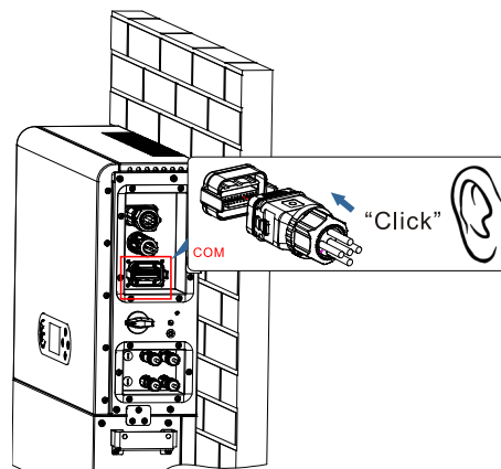
Figura 42 - Collegamento COM
