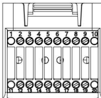
Figura 37 - Schema della porta COM
