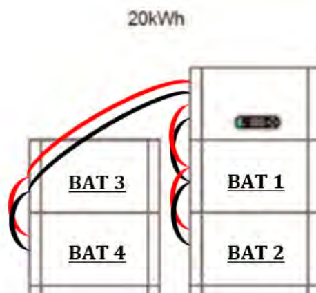
Figura 22 - Collegamento del terminale DC interno della batteria (doppia colonna)
