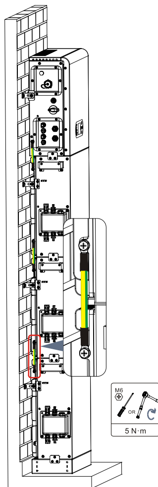
Figura 16- Collegamento di messa a terra interno
