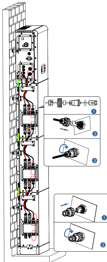
Figura 18 - Collegamento del cavo del segnale interno
