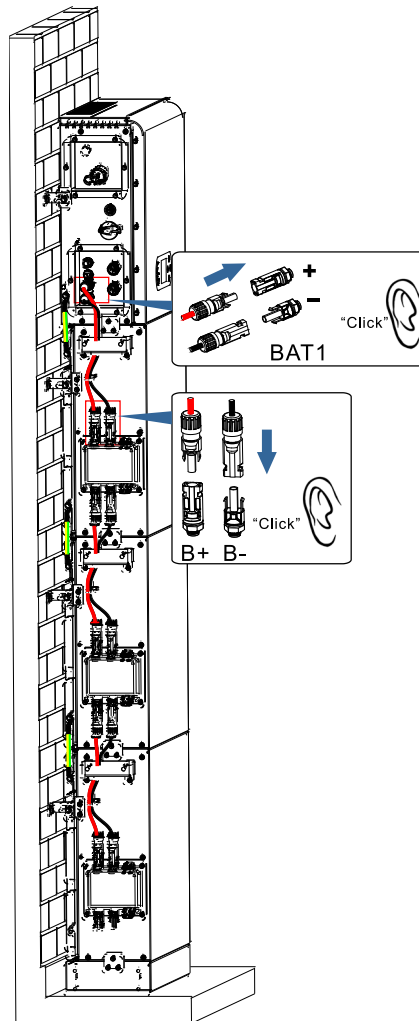
Figura 17 - Collegamento del terminale DC interno della batteria
