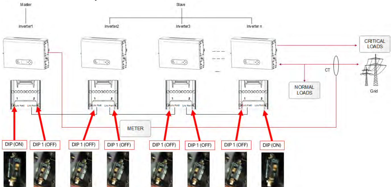
Figura 53- Diagramma del sistema parallelo
