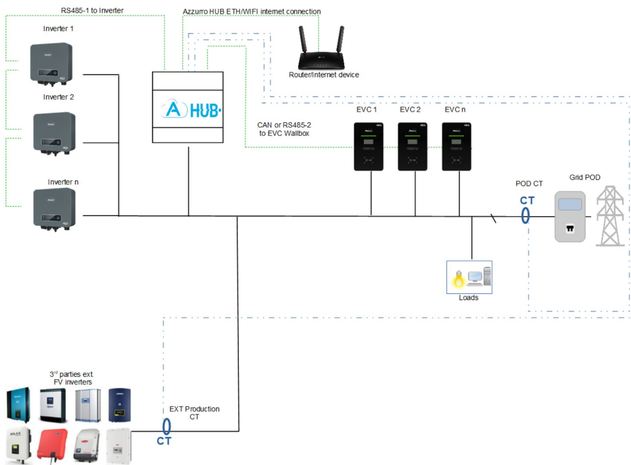
Figura 9 - Schema Impianto SENSORI collegati direttamente all'Azzurro HUB
