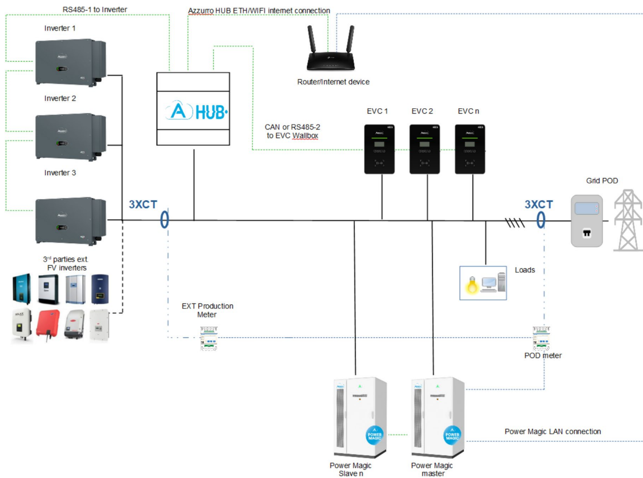
Figura 8 - Schema Impianto POWER MAGIC
