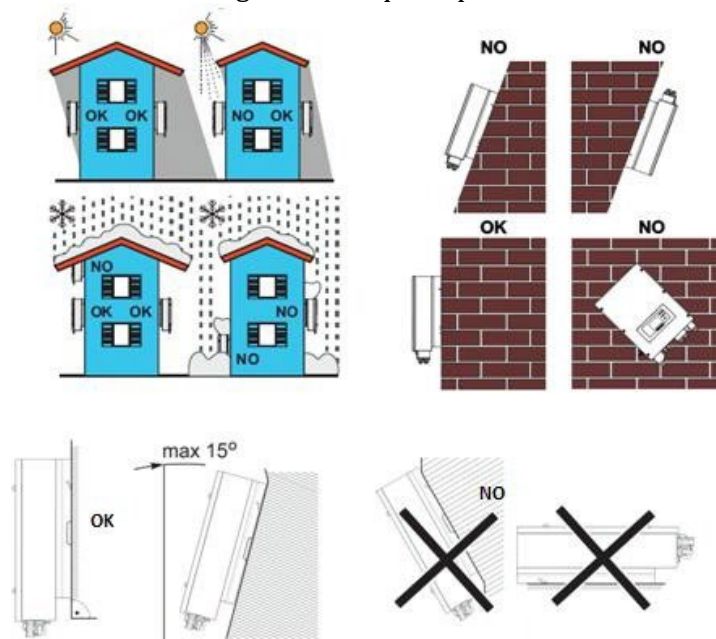
Figura 4 - Posición de instalación del inversor 1PH HYD3000-HYD6000-ZSS
