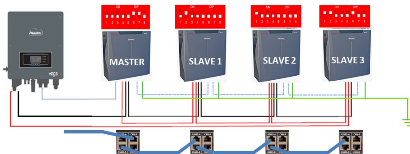
Figura 31 - Paralelo de cuatro baterías WeCo 5k3
