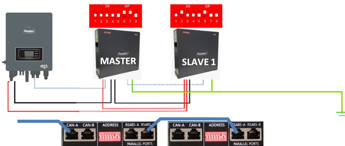
Figura 22 – Paralelo de dos baterías WeCo 4k4 PRO
