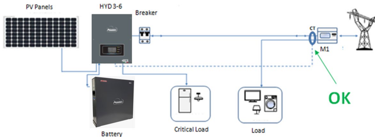
Figura 63 – Posicionamiento correcto de las sondas de corriente para instalación con dos líneas separadas
