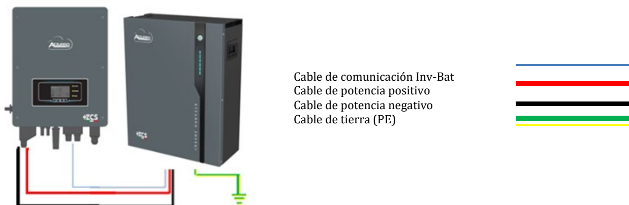
Figura 45- Conexión de la batería AZZURRO 5000
