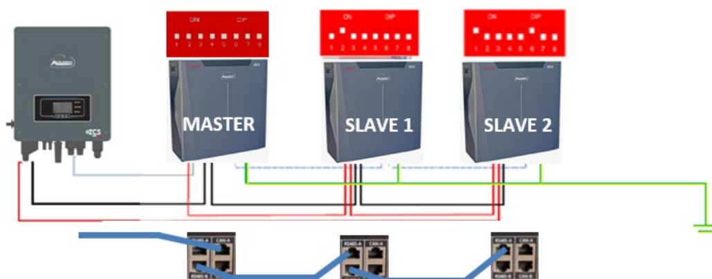
Figura 41 - Conexión en paralelo con 5K3XP Master y 5K3 Slave
