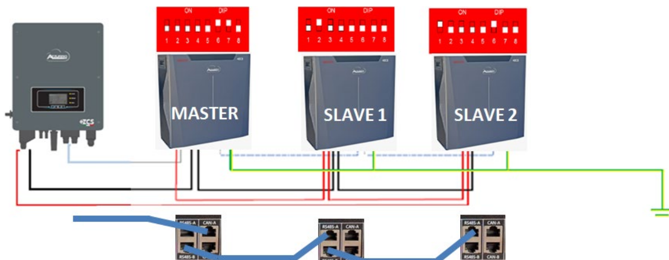
Figura 30 - Paralelo de tres baterías WeCo 5k3
