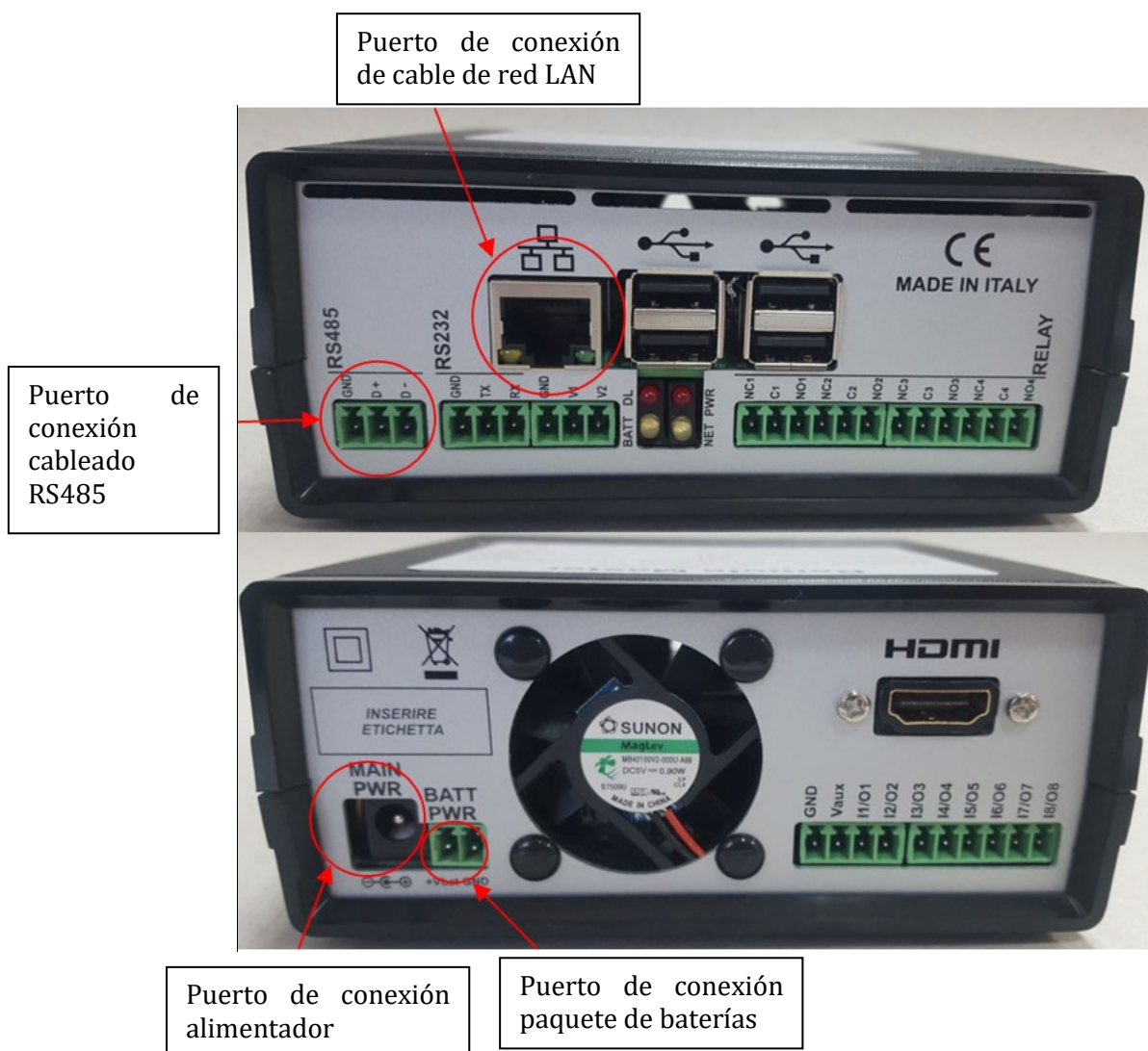
Figura 142: Trasera del Datalogger
