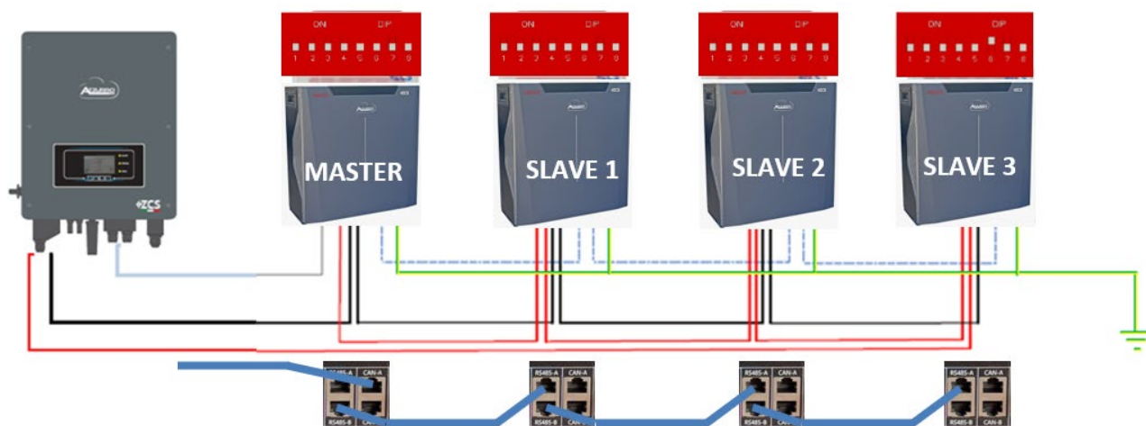
Figura 38 – Conexión en paralelo de cuatro baterías WeCo 5K3XP
