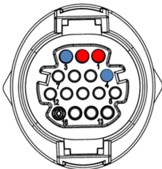
Figura 122a- Conexión de la línea serie mediante conector de comunicación para 3PH HYD5000-HYD20000-ZSS
