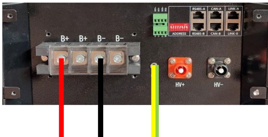
Figura 27- Conexión de la batería WeCo 5k3
