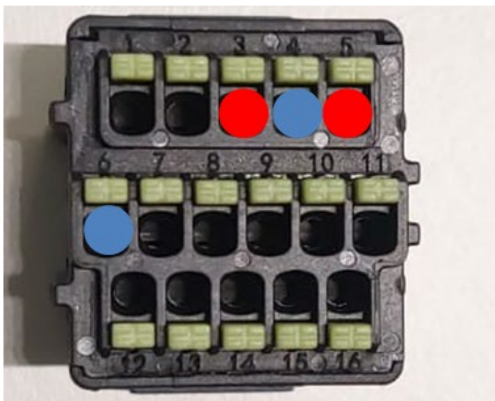
Figura 122c- Conexión de la línea serie mediante conector de comunicación para 1PH HYD3000- ZSS-HP
