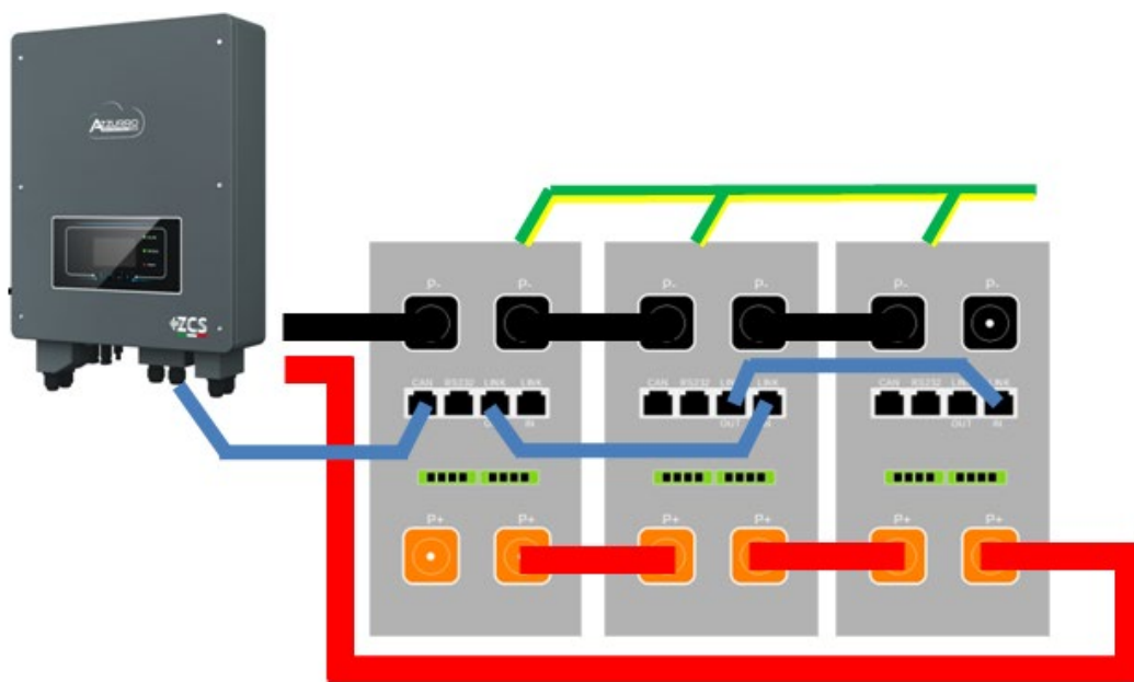
Figura 50 – Paralelo de tres baterías AZZURRO 5000
