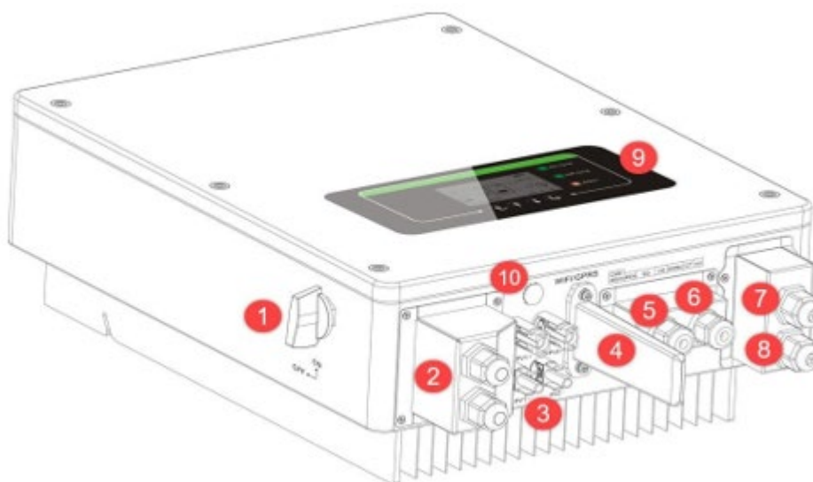
Figura 2- Diagrama en esquema de un equipo en que se ha instalado un inversor híbrido 1PH HYD3000-HYD6000-ZSS
