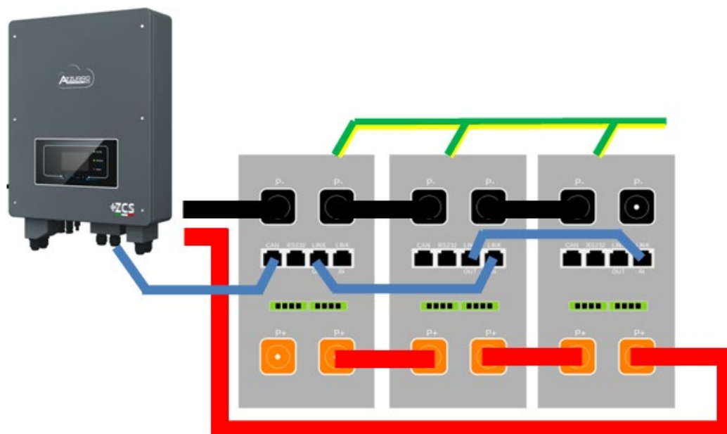
Figura 50 – Paralelo de tres baterías AZZURRO 5000 PRO
