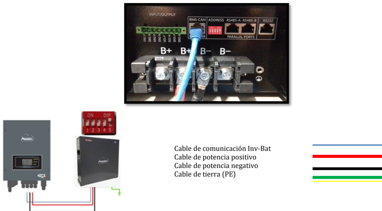
Figura 13- Conexión de la batería WeCo 4k4
