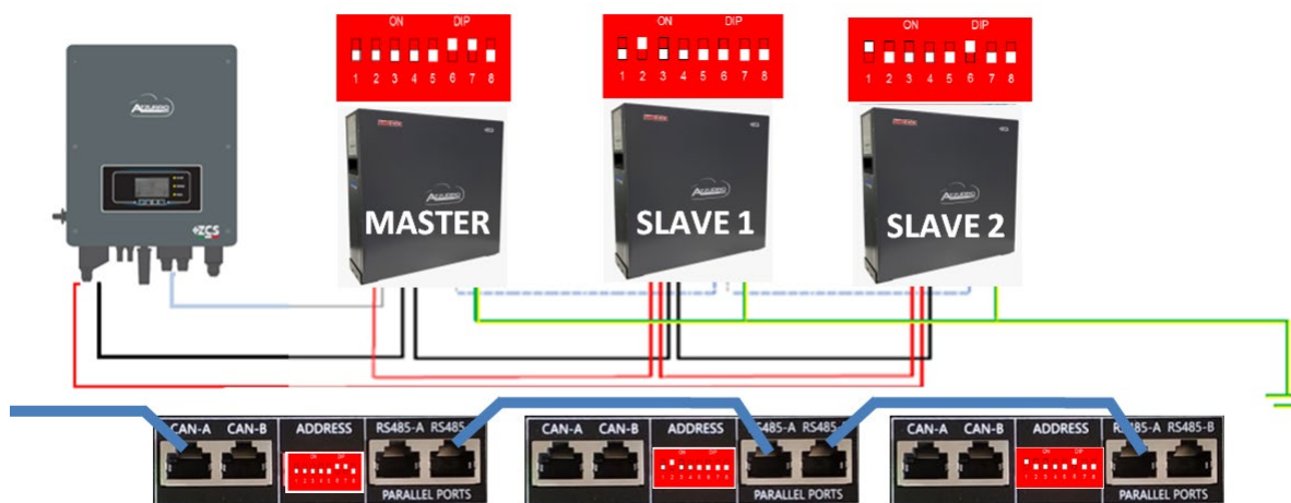
Figura 23 – Paralelo de tres baterías WeCo 4k4 PRO
