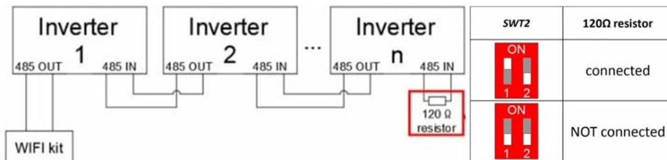
Figura 123 – Posición de los interruptores dip para conectar la resistencia de aislamiento
