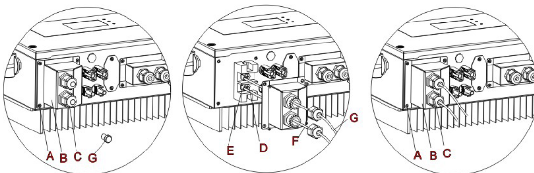
Figura 7- Conexión de la batería (Medir polaridad/voltaje de los cables de la batería antes de la conexión)
