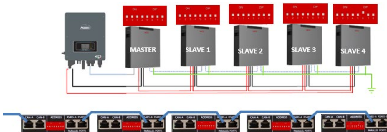
Figura 10 – Conexión en paralelo de cinco baterías WeCo 4k4-LT
