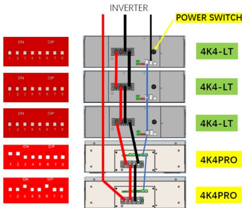
Figura 11 – Conexión en BATERÍAS Weco 4k4-LT y 4k4 PRO
