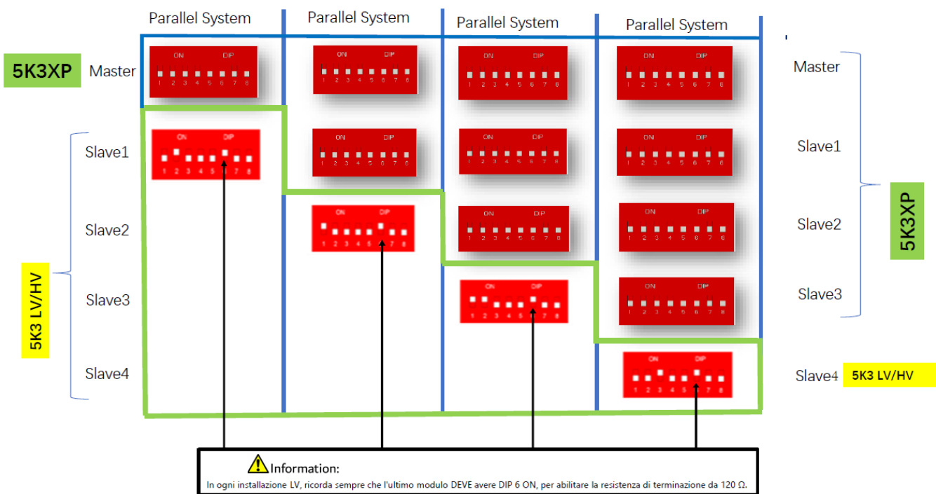
Figura 42 – Colegiado en paralelo a WeCo 5K3XP y WeCo 5K3X (esempio 2)
