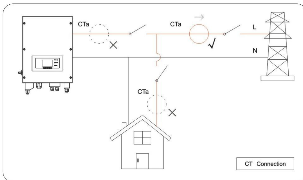
Figura 57 - Conexiones CT
