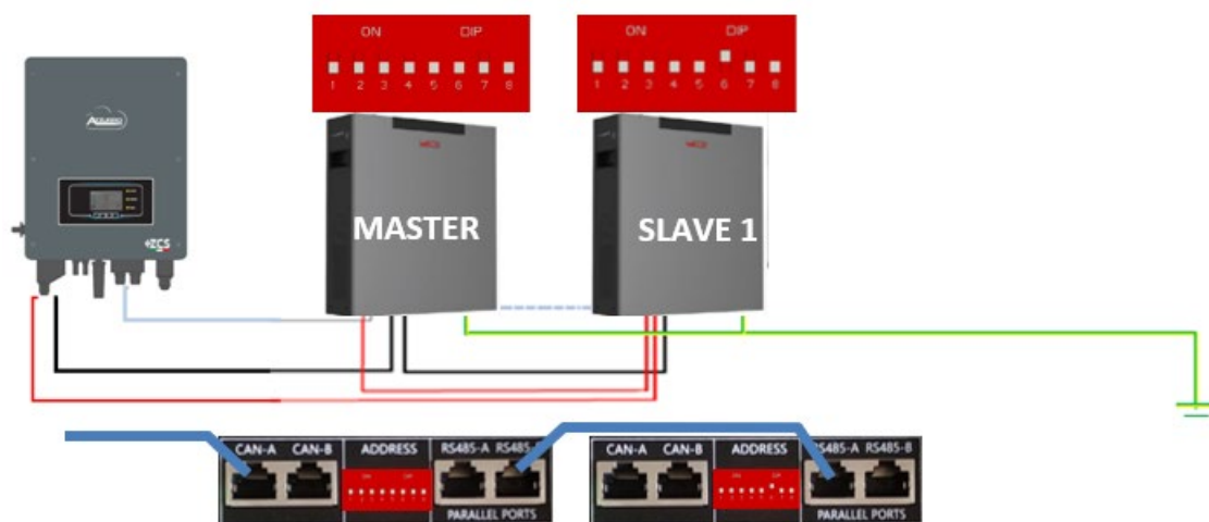
Figura 7 – Conexión en paralelo de dos baterías WeCo 4k4-LT
