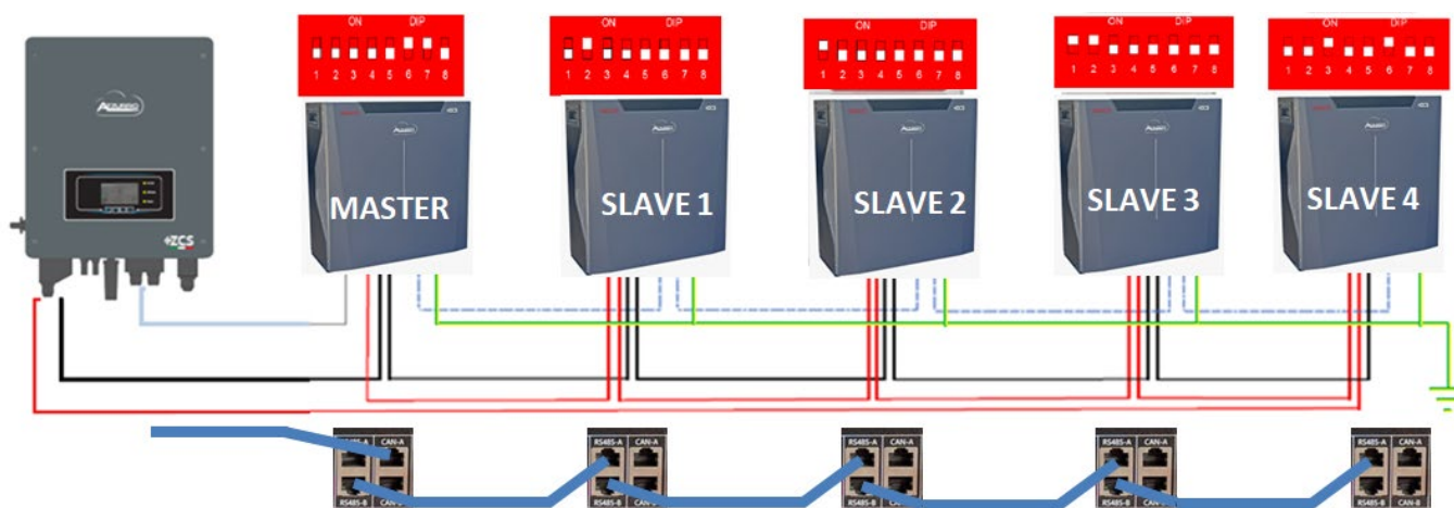
Figura 32 - Paralelo de cinco baterías WeCo 5k3
