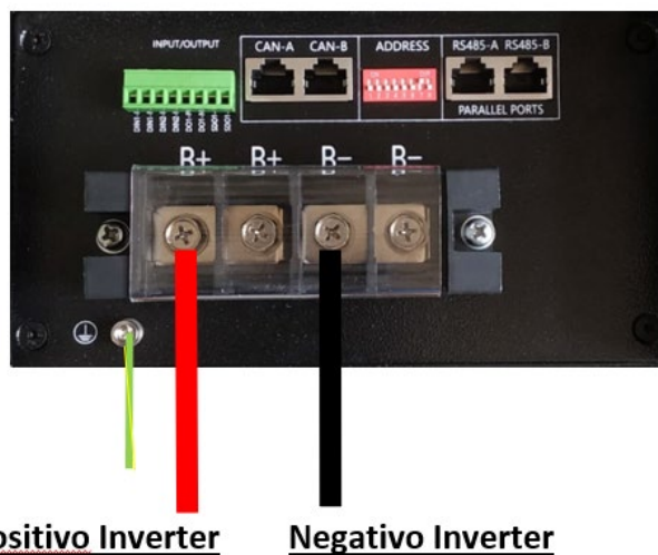
Figura 5- Conexión del cable de potencia de la batería Weco 4k4-LT al inversor
