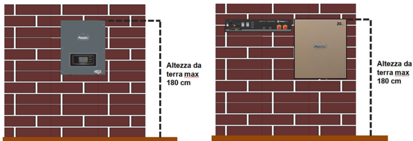
Figura 5 – Indicaciones para la instalación del inversor de acumulación y del paquete de baterías
