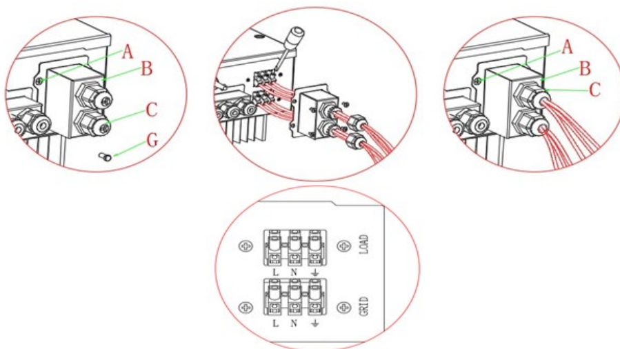
Figura 64– Conexión de red y cargas críticas.
