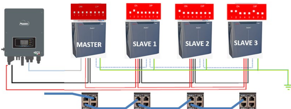
Figura 42 - Conexión en paralelo con 5K3XP Master y 5K3 Slave
