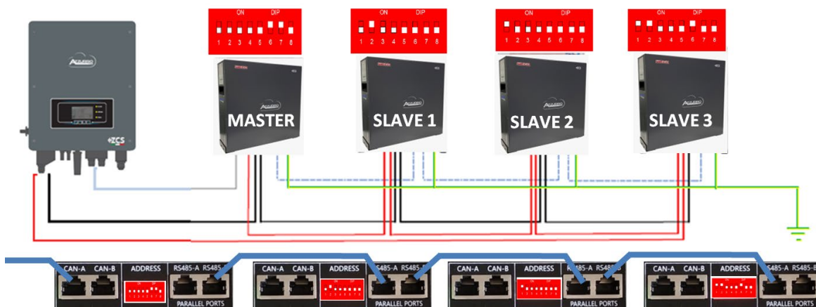
Figura 24 – Paralelo de cuatro baterías WeCo 4k4 PRO
