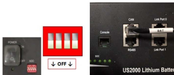
Figura 9 - Conexión del cable de comunicación en la batería Pylontech
