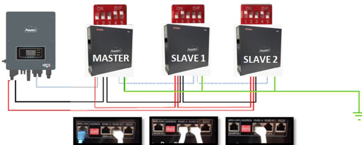
Figura 16 – Paralelo de tres baterías WeCo 4k4
