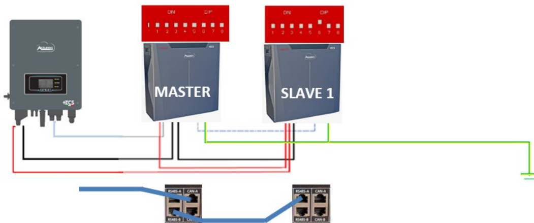
Figura 36 – Conexión en paralelo de dos baterías WeCo 5K3XP
