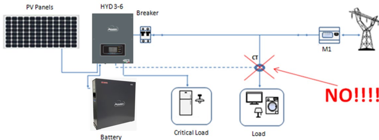
Figura 62 – Colocación errónea de las sondas de corriente (Lectura Cta únicamente de los dispositivos usuarios)
