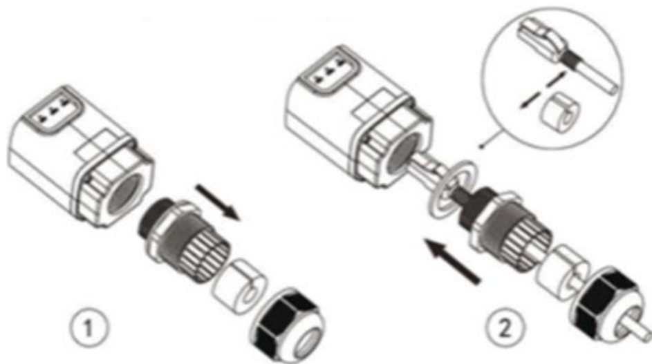
Figura 106 – Introducción del cable de red en el dispositivo
