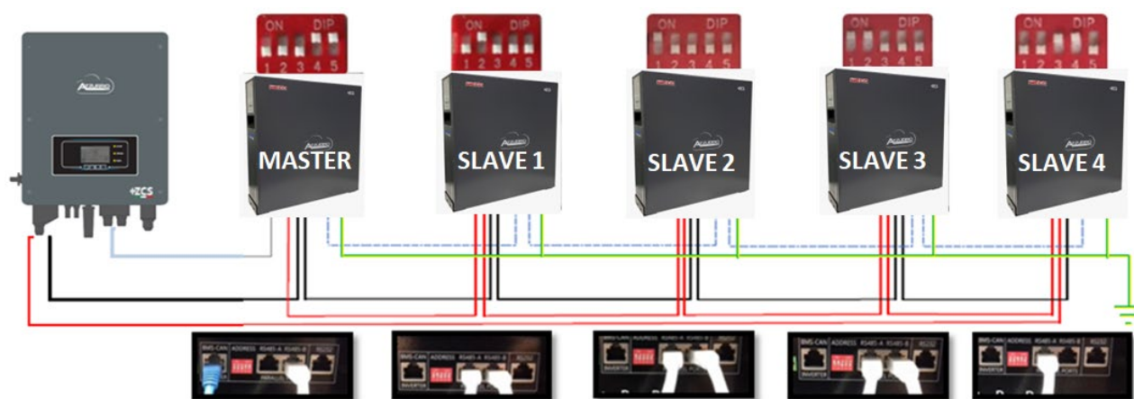
Figura 18 - Paralelo de cinco baterías WeCo 4k4
