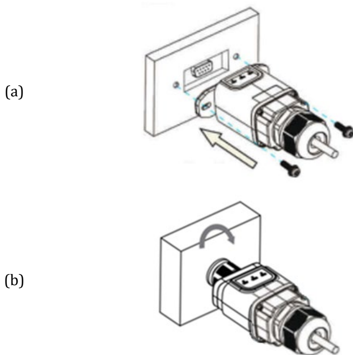
Figura 88 – Introducción y fijación de la tarjeta ethernet
