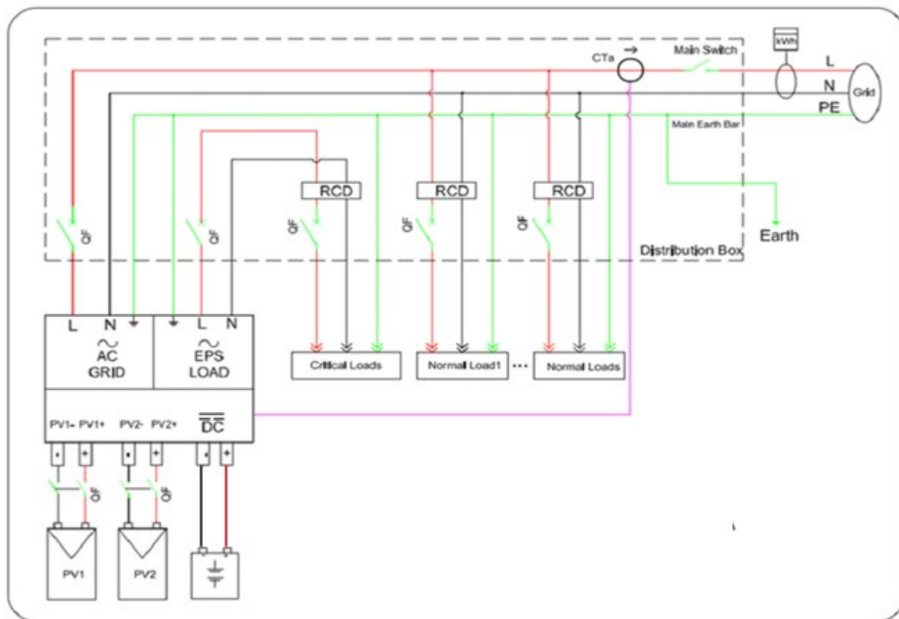
Figura 6- Conexiones eléctricas
