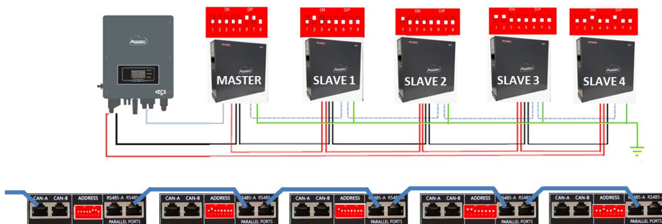
Figura 25 – Paralelo de cinco baterías WeCo 4k4 PRO
