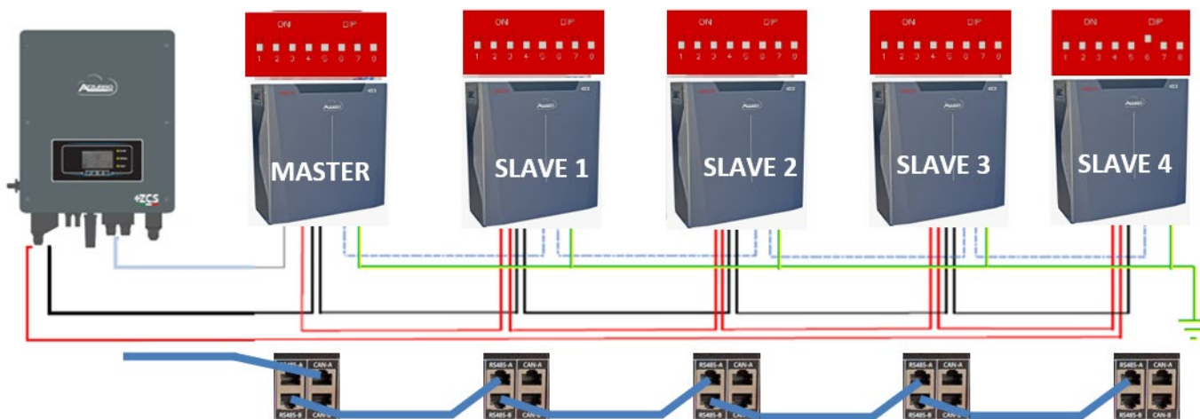
Figura 39 – Conexión en paralelo de cinco baterías WeCo 5K3XP
