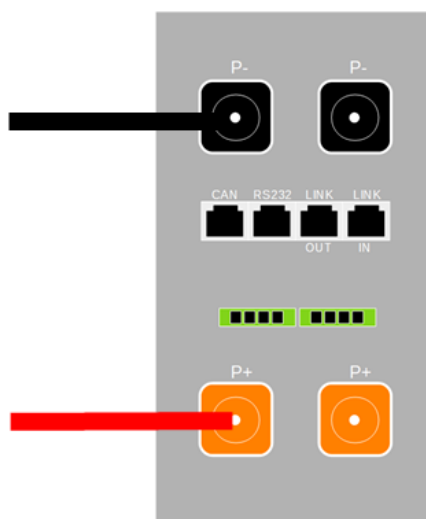
Figura 46- Conexiones de la batería AZZURRO 5000
