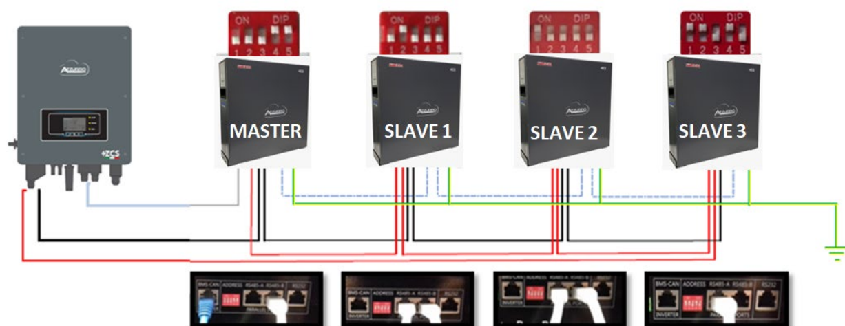
Figura 17 - Paralelo de cuatro baterías WeCo 4k4
