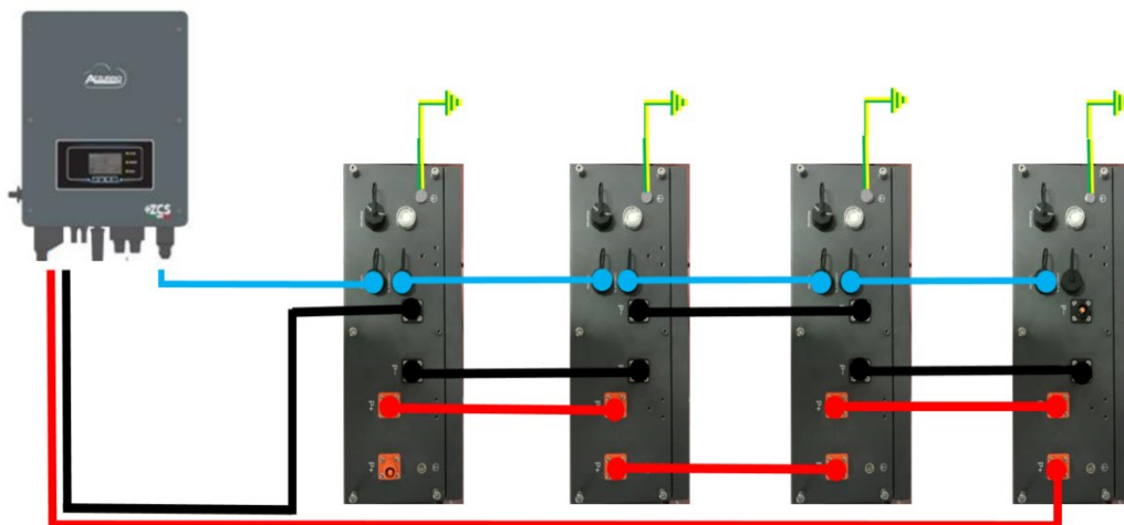
Figura 53 – Paralelo de cuatro baterías AZZURRO ZSX 5000S
