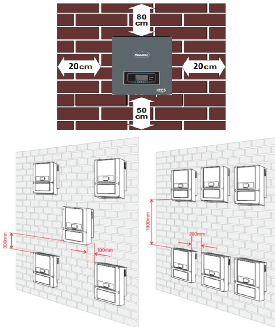
Figura 4 - Posición de instalación del inversor 1PH HYD3000-HYD6000-ZSS
