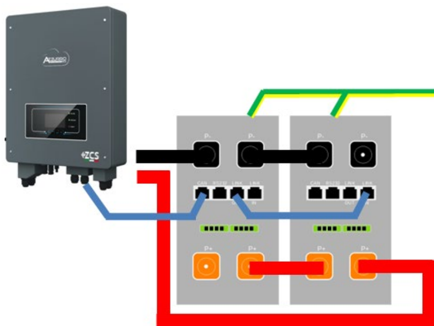
Figura 49 – Paralelo de dos baterías AZZURRO 5000 PRO
