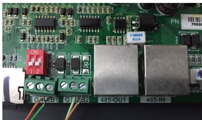
Figura 121 - Conexión de línea serie mediante regleta RS485 y mediante clavija RJ45
