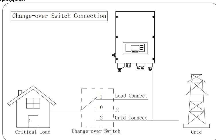
Figura 65– Conexiones del conmutador
