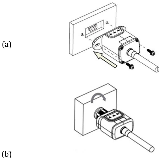
Figura 113 - Introducción y fijación de la tarjeta 4G
