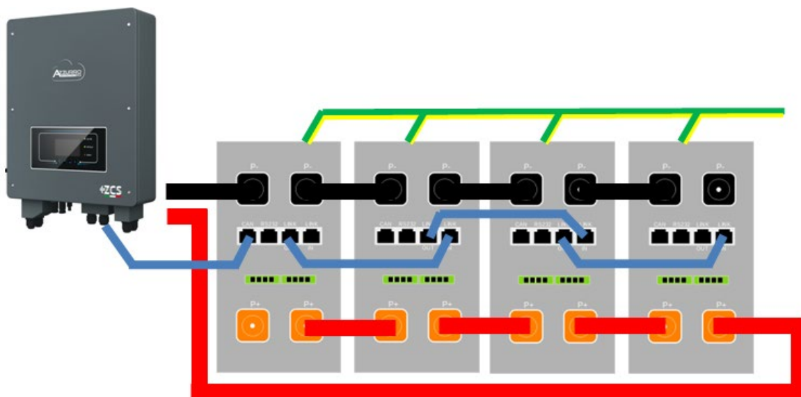
Figura 51 – Paralelo de cuatro baterías AZZURRO 5000
