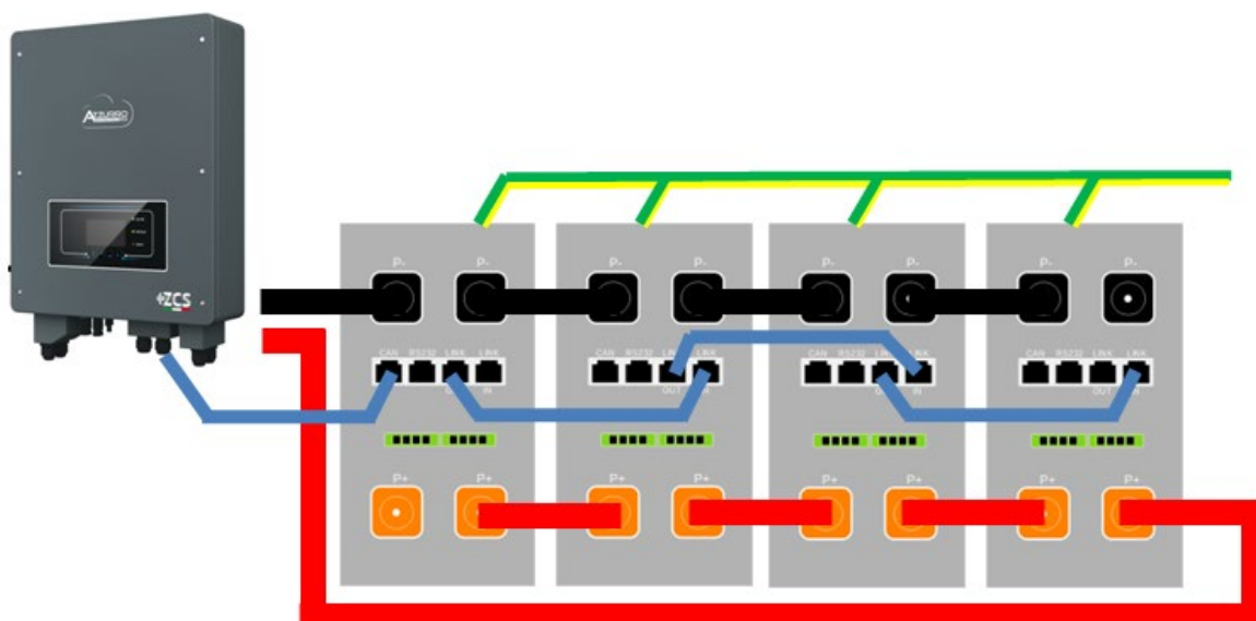
Figura 51 – Paralelo de cuatro baterías AZZURRO 5000 PRO
