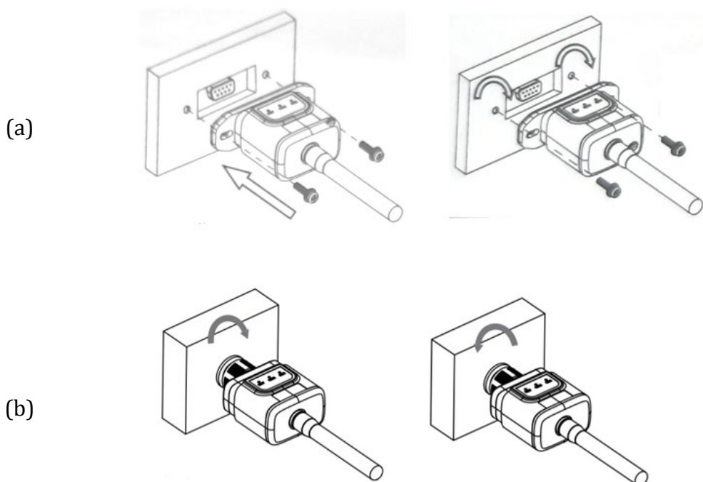
Figura 81 – Introducción y fijación de la tarjeta wifi externa
