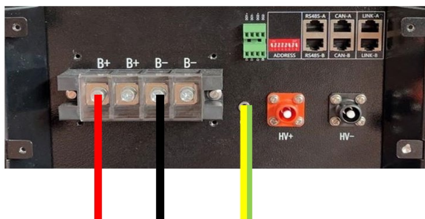
Figura 34- Conexión de la batería WeCo 5K3XP
