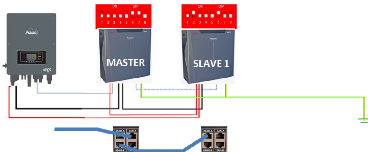
Figura 29 – Paralelo de dos baterías WeCo 5k3
