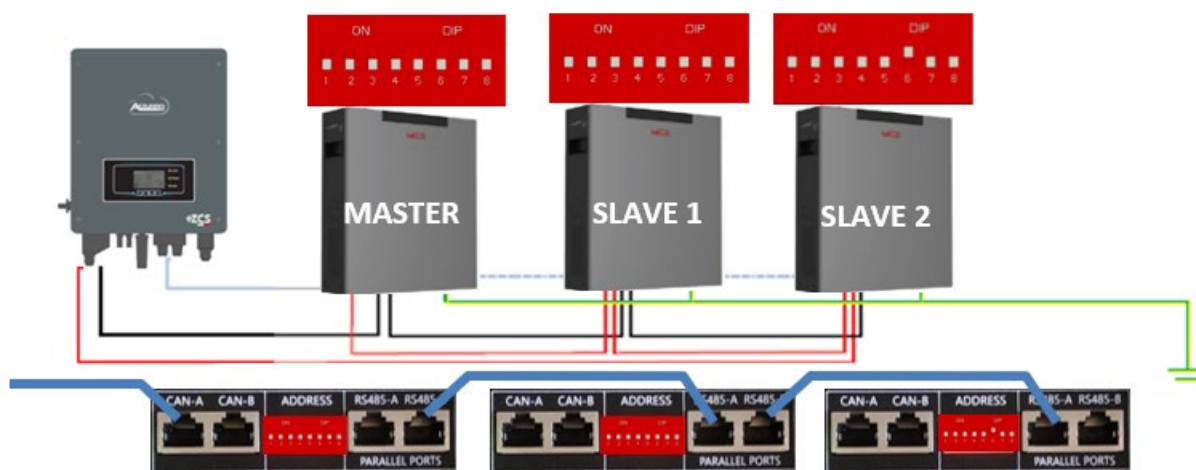
Figura 8 – Conexión en paralelo de tres baterías WeCo 4k4-LT
