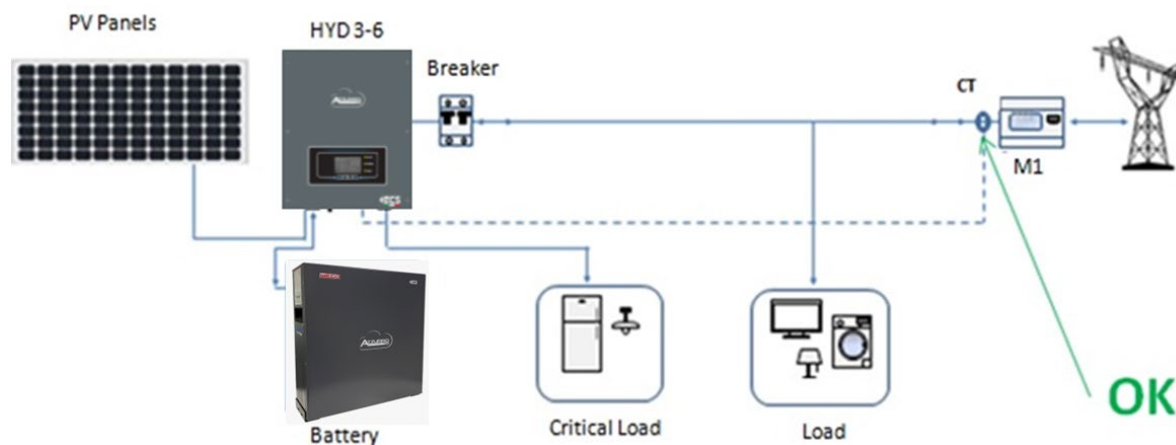
Figura 61 – Posicionamiento correcto de las sondas de corriente
