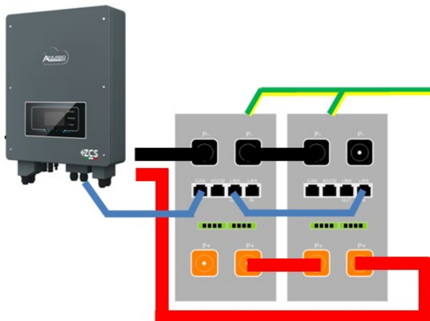
Figura 49 – Paralelo de dos baterías AZZURRO 5000
