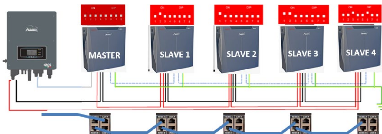
Figura 43 - Conexión en paralelo con 5K3XP Master y 5K3 Slave
