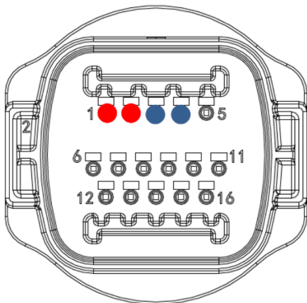
Figura 122b- Conexión de la línea serie mediante conector de comunicación para 3PH HYD5000-HYD20000-ZSS y 3000-6000 TLM-V3
