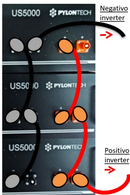
Figura 30 - Paralelo de tres baterías Pylontech
