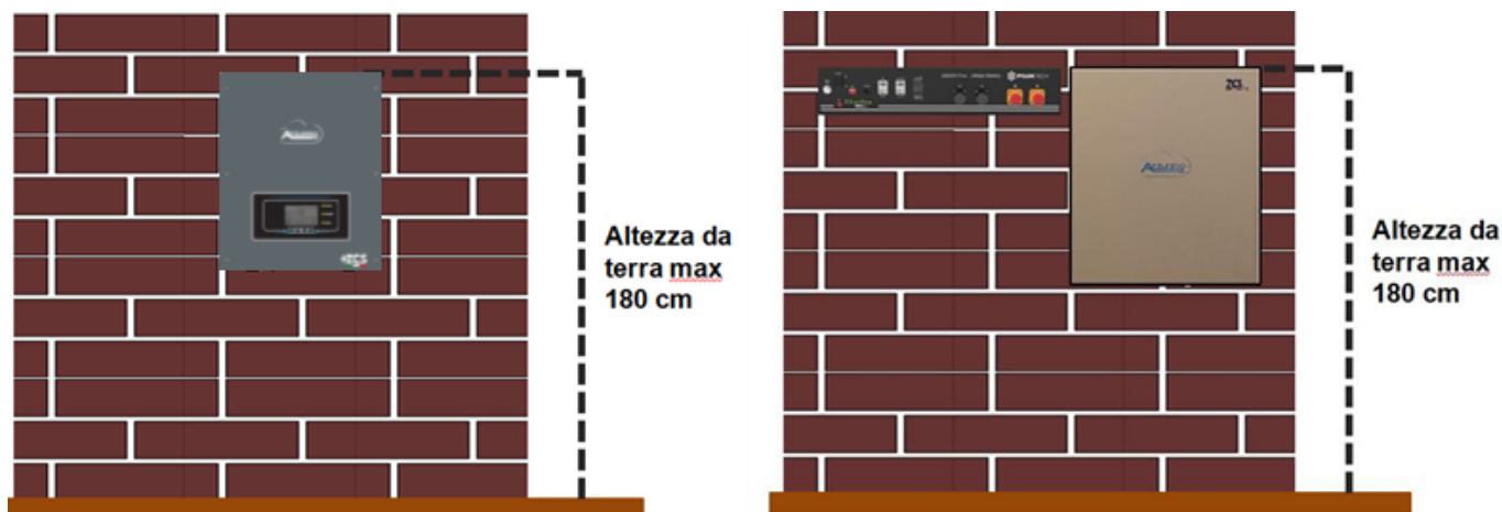
Figure 5 – Instructions pour l'installation de l'onduleur de stockage et du pack batterie
