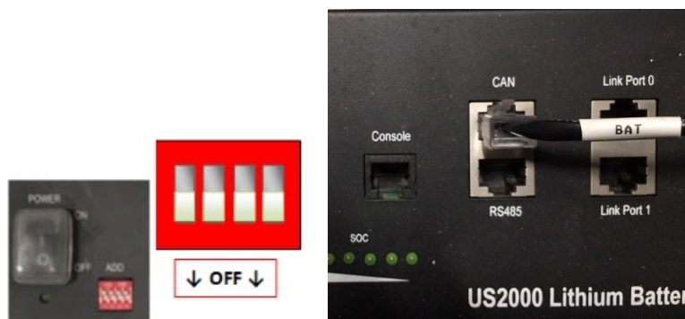
Figure 9 – Connexion du câble de communication sur la batterie Pylontech
