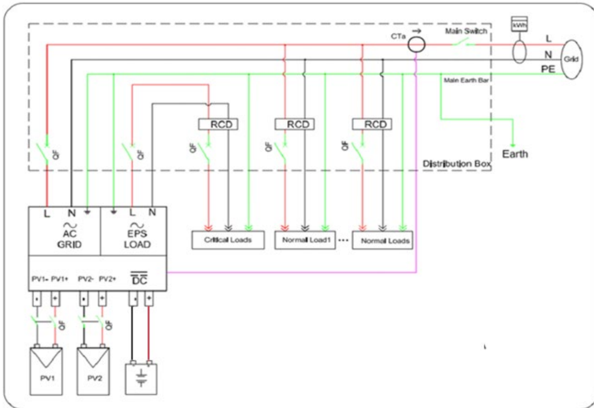
Figure 6 – Raccordements électriques
