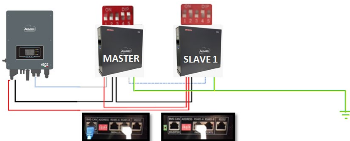
Figure 15 – Parallèle de deux batteries WeCo 4k4
