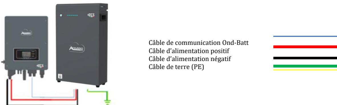
Figure 48 - Connexion de la batterie AZZURRO ZSX 5000 S
