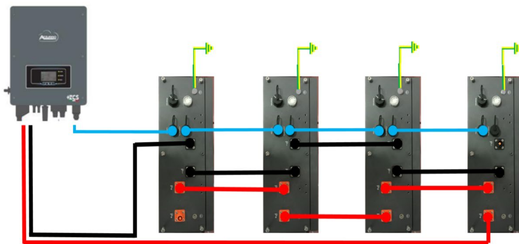
Figure 53 – Parallèle de quatre batteries AZZURRO ZSX 5000 S
