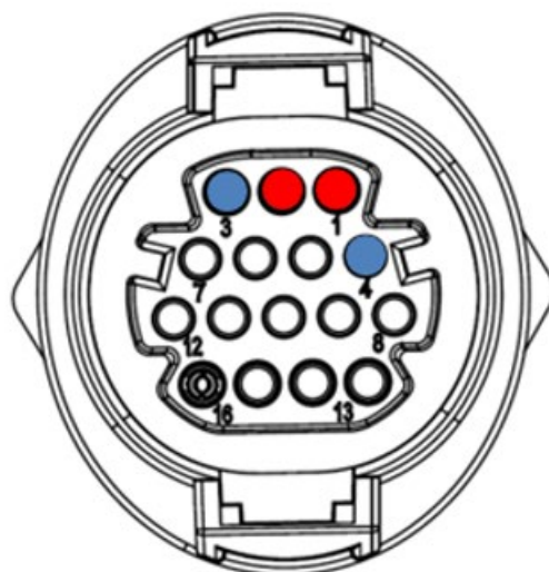
Figure 117a- Connexion ligne série via connecteur de communication pour 3PH HYD5000-HYD20000-ZSS
