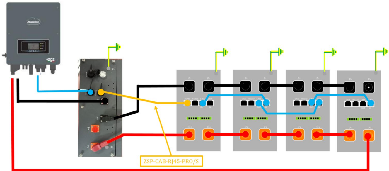
Figure 14 – Connexion en parallèle de la batterie AZZURRO 5000S et AZZURRO 5000/AZZURRO 5000PRO
