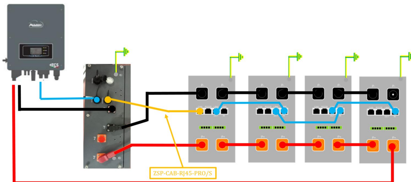
Bild 86 - Parallelschaltung von AZZURRO 5000S und AZZURRO 5000/AZZURRO 5000PRO
