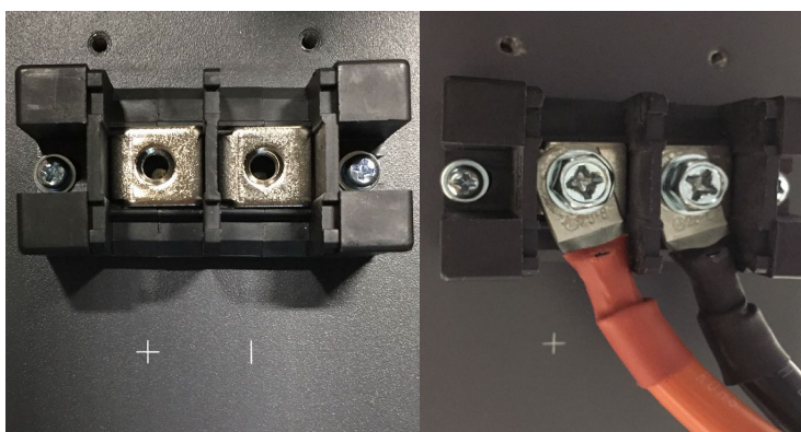
Abbildung 10 - Stromanschluss der Batterie
