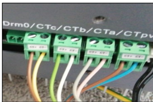
Abbildung 78- Anschlüsse der CT-Kabel für die Stromsonden
