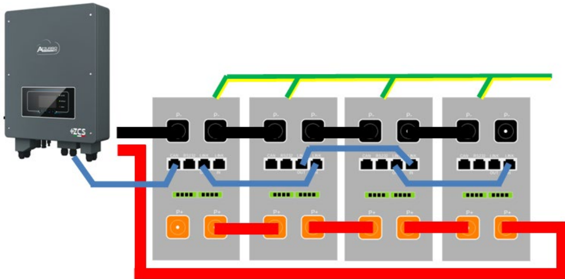
Abbildung 54 – Parallelverbindung von vier Batterien AZZURRO ZSX 5120
