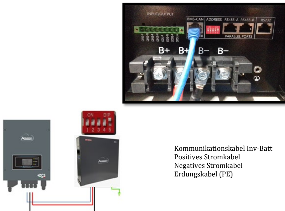
Abbildung 16 - Anschluss WeCo Batterie 4K4
