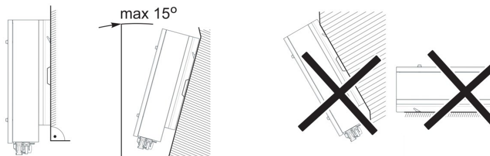
Abbildung 5 - Richtige Installationsstellung des Inverters 3000SP
