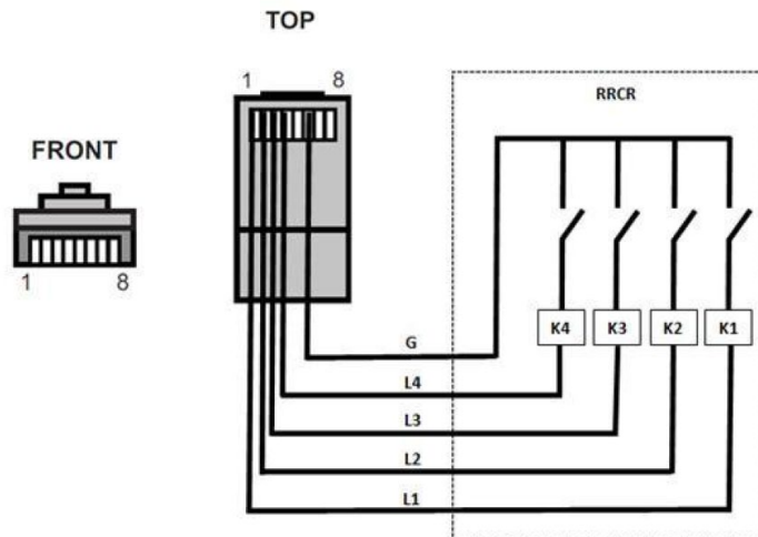
Abbildung 54 – Inverter - RRRC Anschluss
