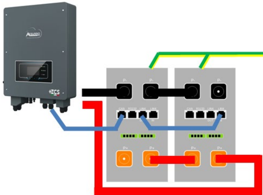
Abbildung 52 – Parallelverbindung von zwei Batterien AZZURRO 5000 PRO
