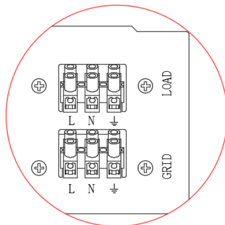
Abbildung 63 - Anschluss des Netzkabels an die Klemmenleiste GRID
