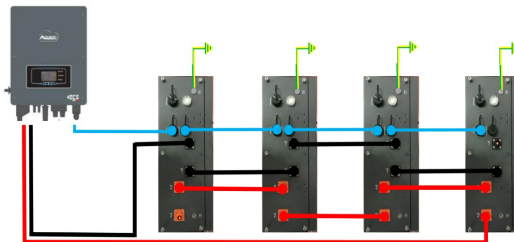
Abbildung 88 – Parallelverbindung von vier Batterien AZZURRO ZSX 5000 S
