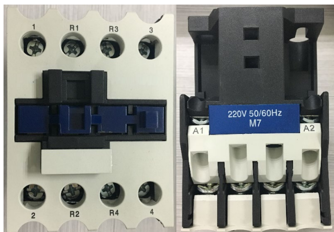
Abbildung 65- Vorderansicht und Aufsicht des Stromkontaktgebers; Anschluss des Kontaktgebers im Inneren der Anlage
