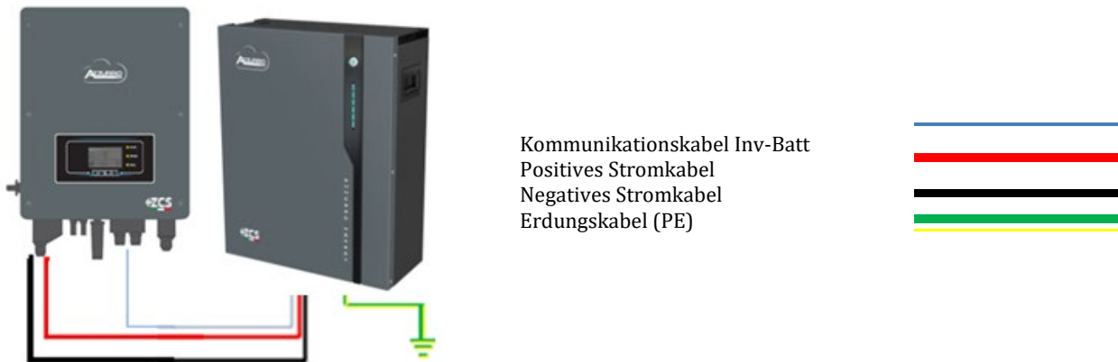
Abbildung 48 - Anschluss Batterie AZZURRO 5000 PRO
