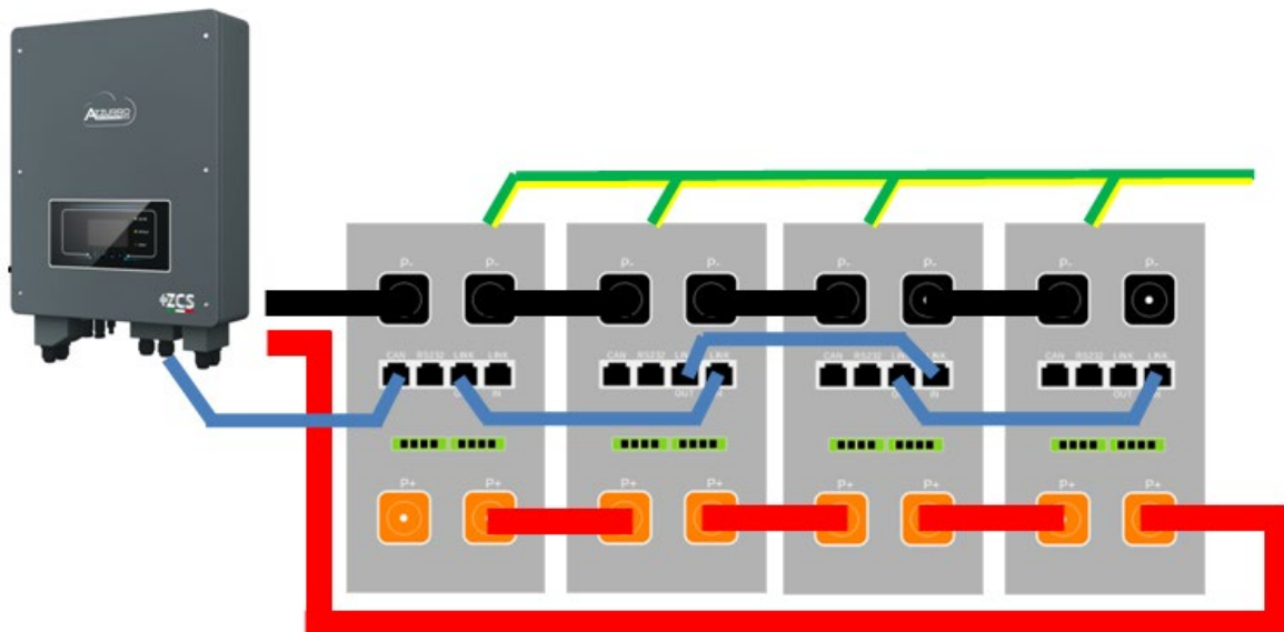
Abbildung 54 – Parallelverbindung von vier Batterien AZZURRO 5000
