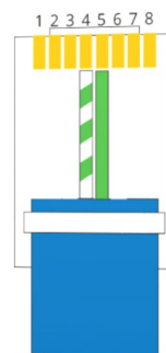
c. Link Out der Slave-Batterie 1 ( 5000/5000 PRO ) → Link In der Slave-Batterie 2 ( 5000/5000 PRO )
