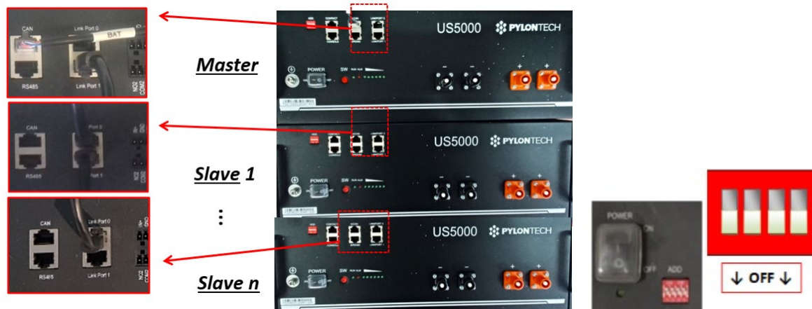
Abbildung 14 – Kommunikationsverbindung zwischen drei Pylontech-Batterien
