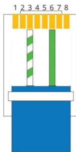
b. CAN der Slave-Batterie 1 (5000/5000 PRO)
