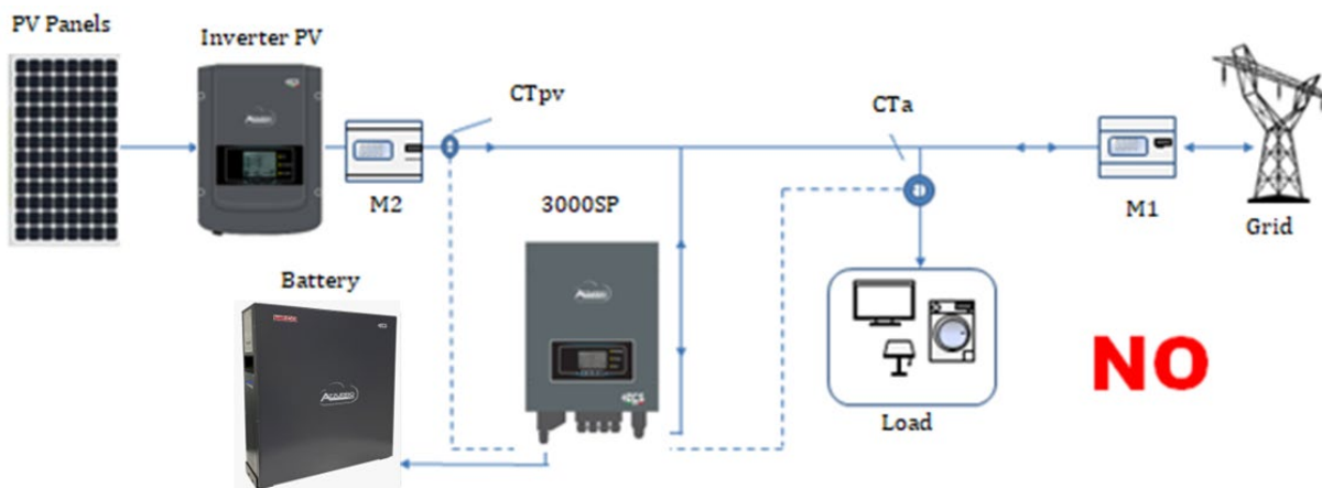
Abbildung 61 – Falsche Positionierung der Stromsonden (Cta-Ablesung nur der Abnehmer)
