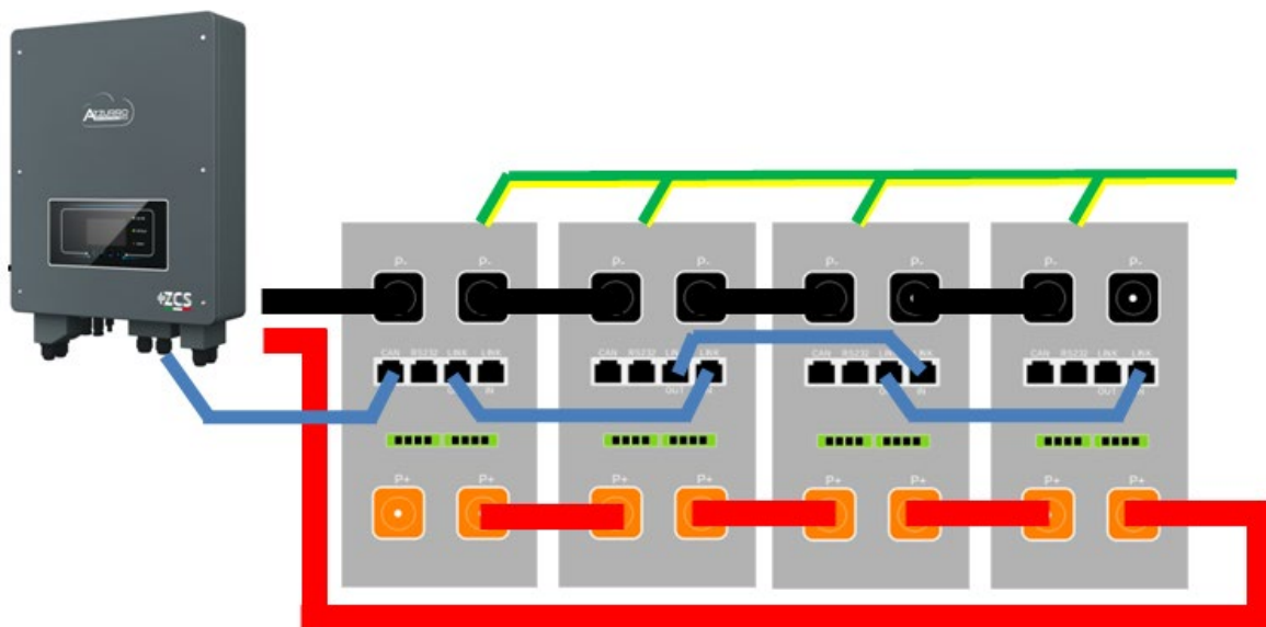
Figure 53 – Parallèle de quatre batteries AZZURRO 5000
