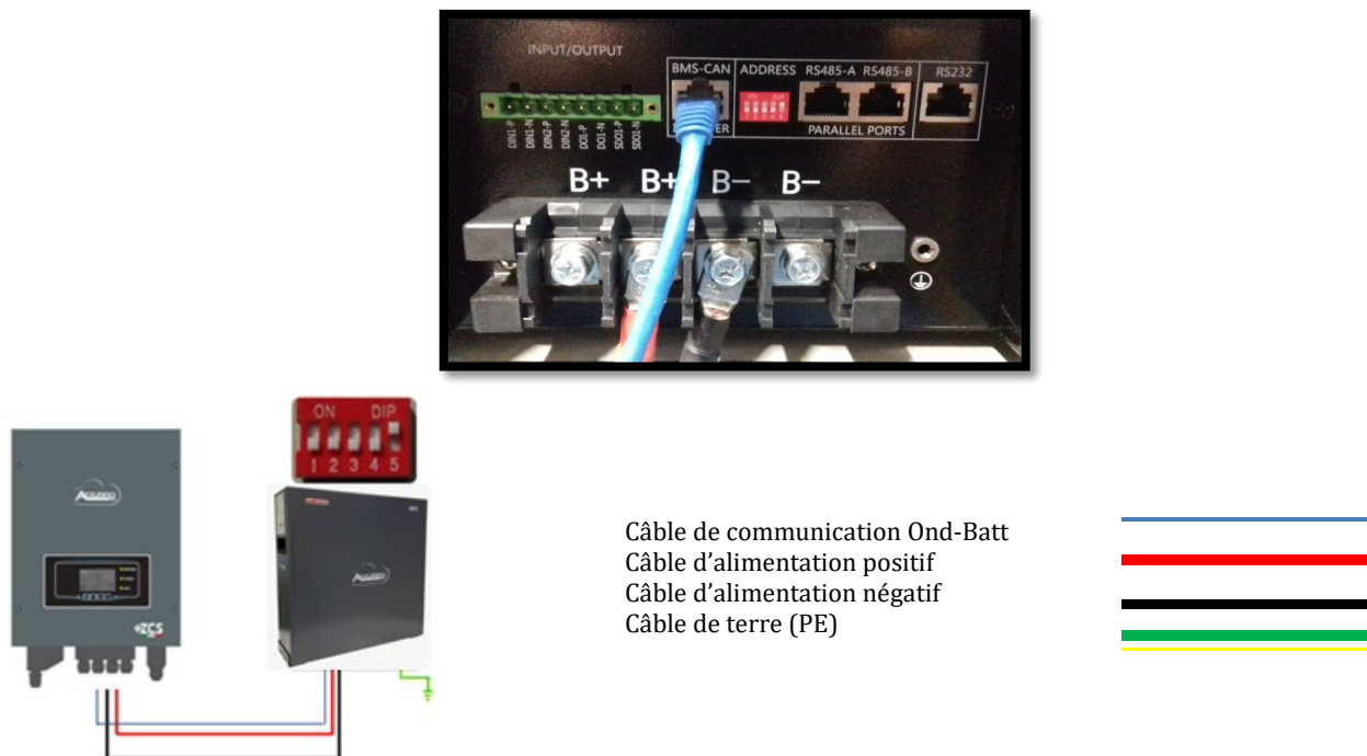
Figure 16 - Connexion de la batterie WeCo 4k4
