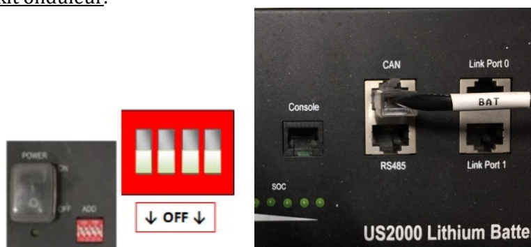
Figure 12 – Connexion du câble de communication sur la batterie Pylontech
