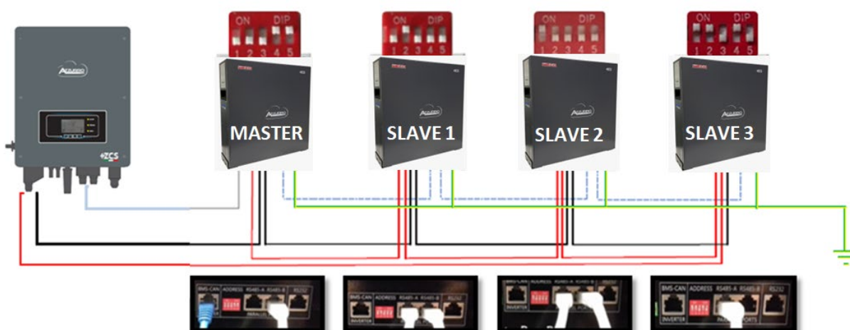
Figure 16 – Parallèle de quatre batteries WeCo 4k4
