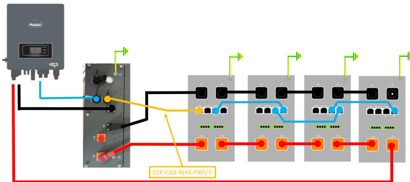
Figure 28 – Connexion en parallèle de la batterie AZZURRO 5000S et AZZURRO 5000/AZZURRO 5000PRO
