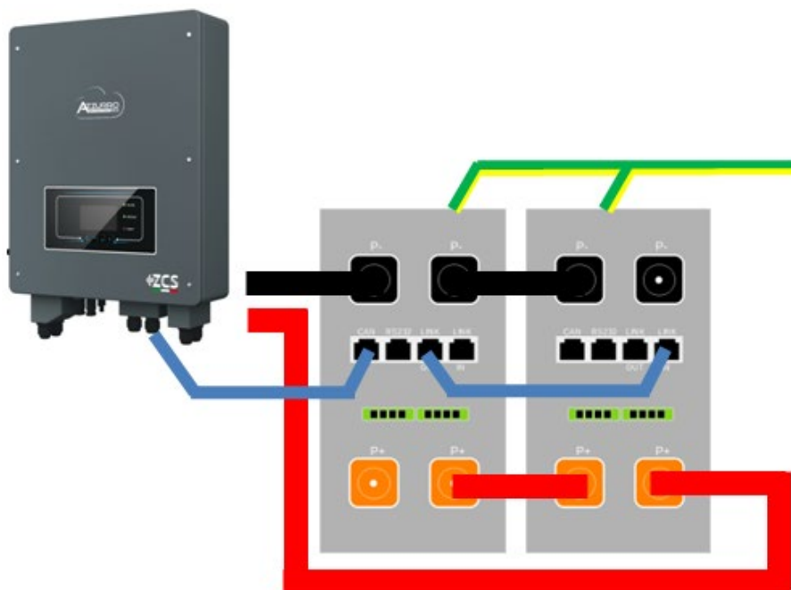
Figure 41 – Parallèle de deux batteries AZZURRO 5000
