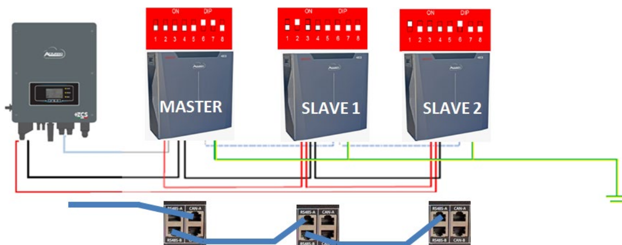
Figure 33 – Parallèle de trois batteries WeCo 5k3
