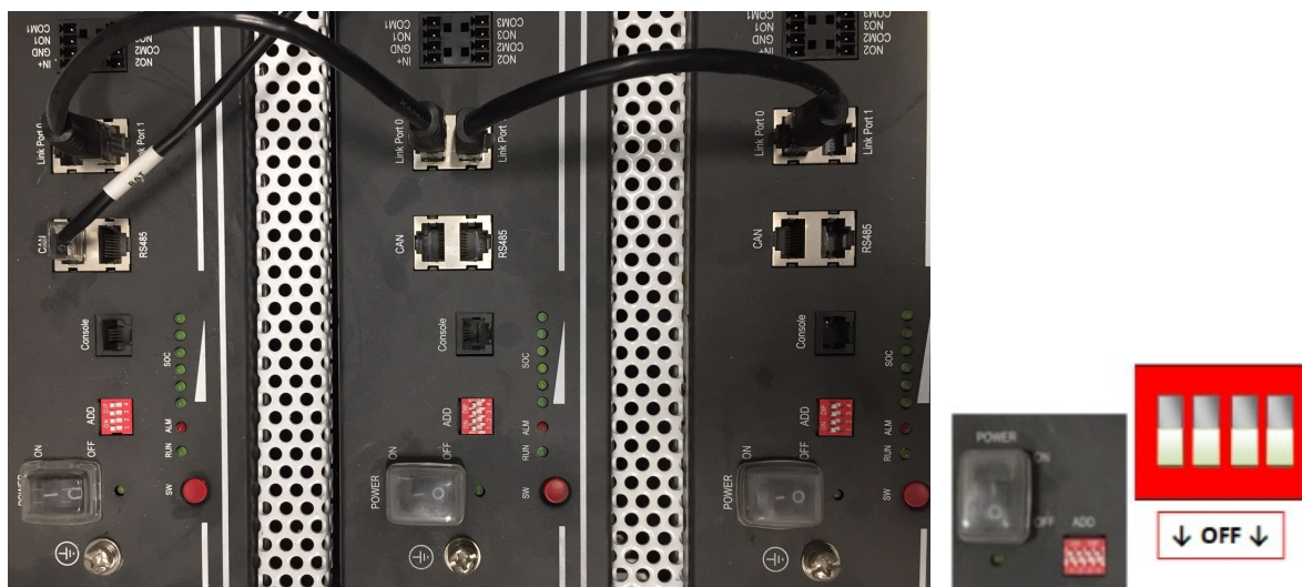
Figure 14 – Connexion de communication entre trois batteries Pylontech
