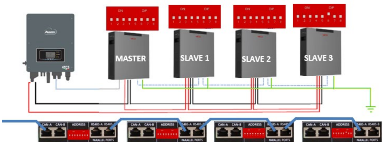
Figure 23 – Connexion en parallèle de quatre batteries WeCo 4k4-LT
