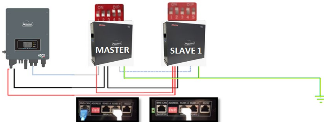
Figure 14 – Parallèle de deux batteries WeCo 4k4
