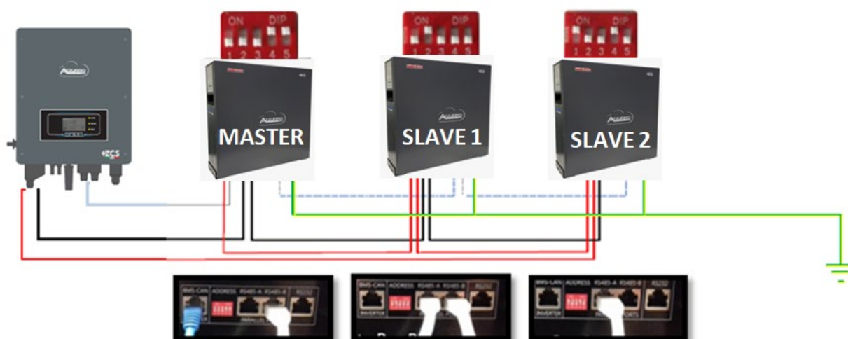
Figure 15 – Parallèle de trois batteries WeCo 4k4
