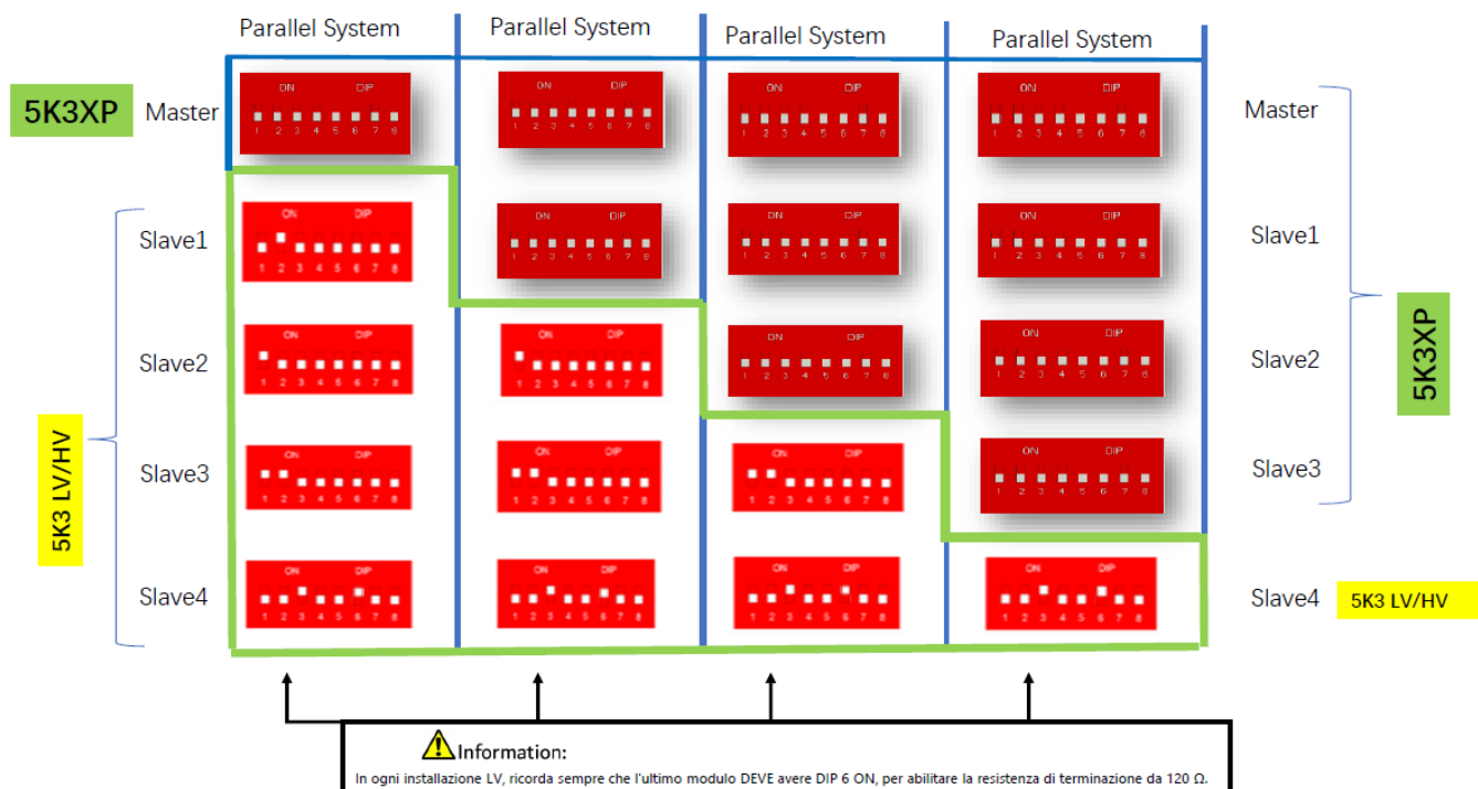
Figura 43 –Connexion en parallèle des batteries WeCo 5K3XP et WeCo 5K3XP (exemple 1)
