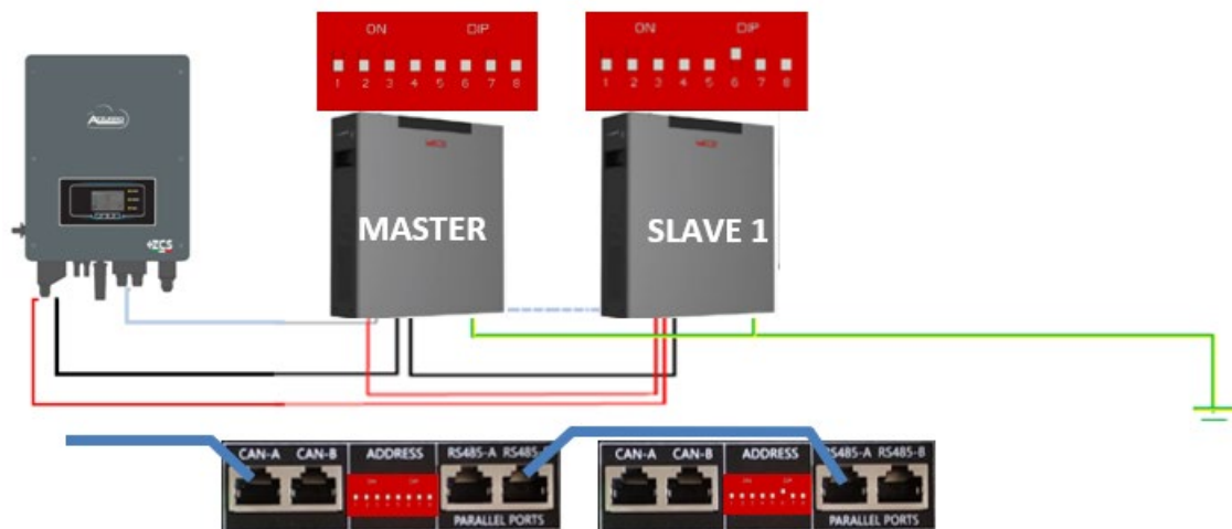
Figure 21 – Connexion en parallèle de deux batteries WeCo 4k4-LT
