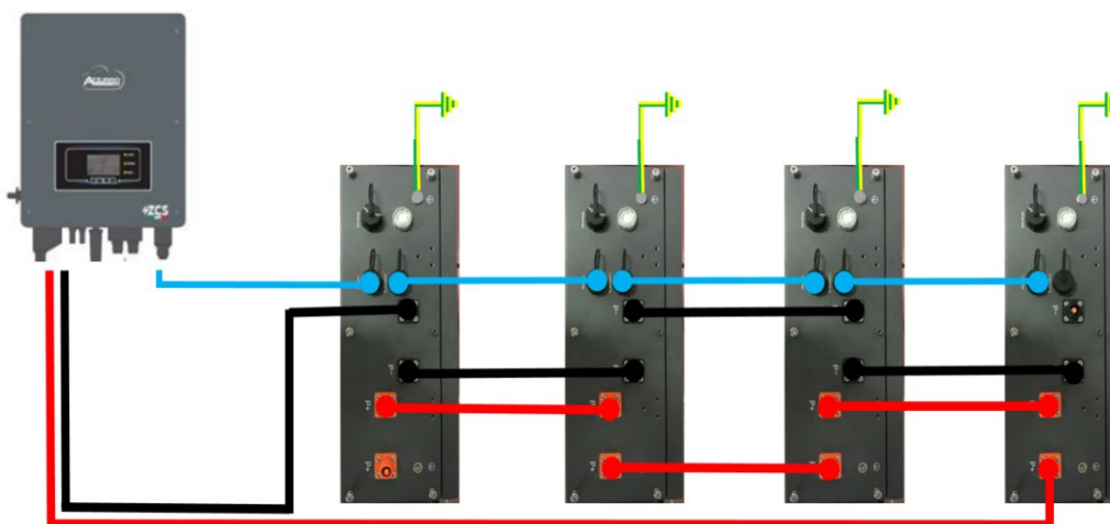
Figure 53 – Parallèle de quatre batteries AZZURRO ZSX 5000 S
