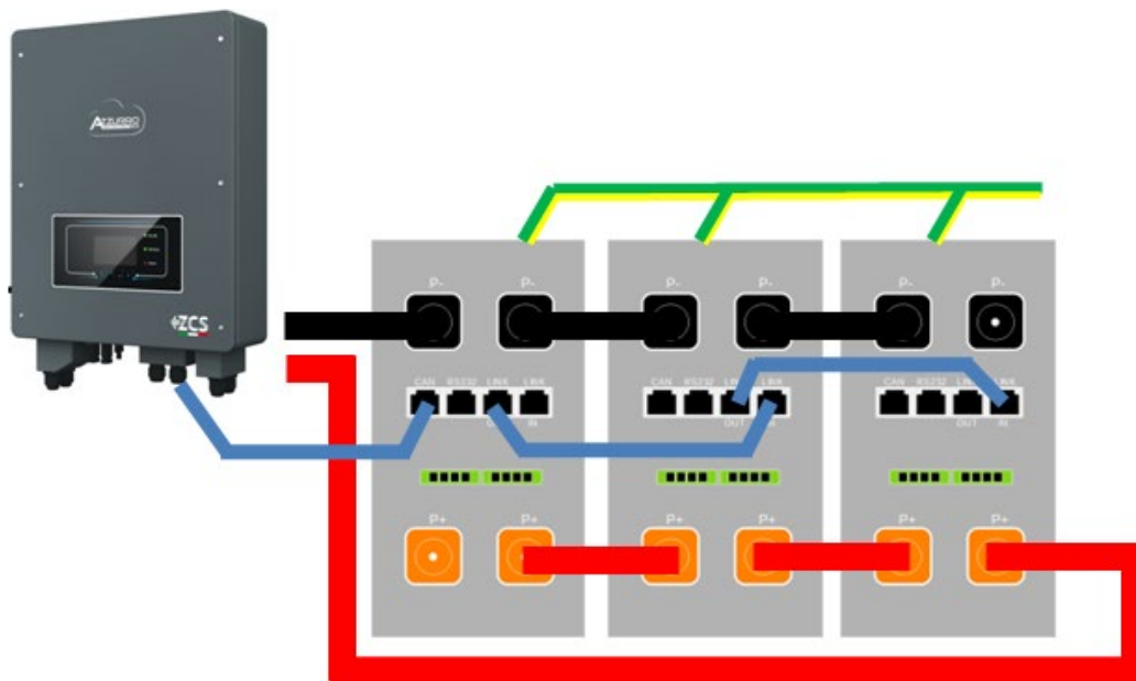
Figure 41 – Parallèle de deux batteries AZZURRO 5000 PRO
