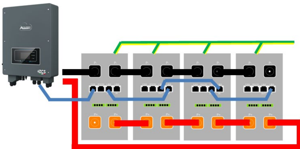
Figure 53 – Parallèle de quatre batteries AZZURRO 5000 PRO
