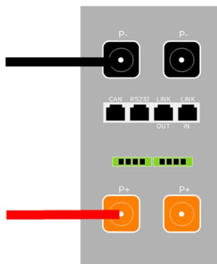
Figure 49 - Bornier batterie AZZURRO 5000 PRO
