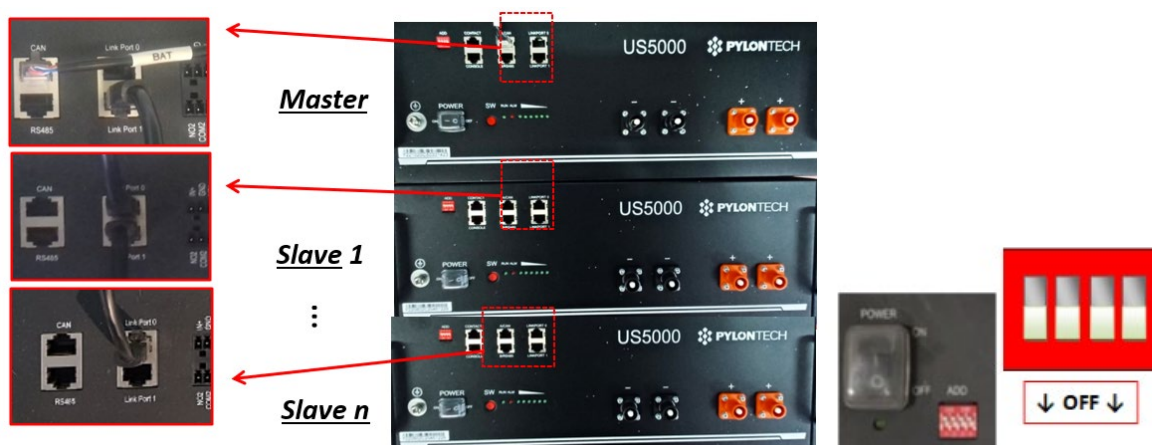
Figure 14 - Connexion de communication entre trois batteries Pylontech
