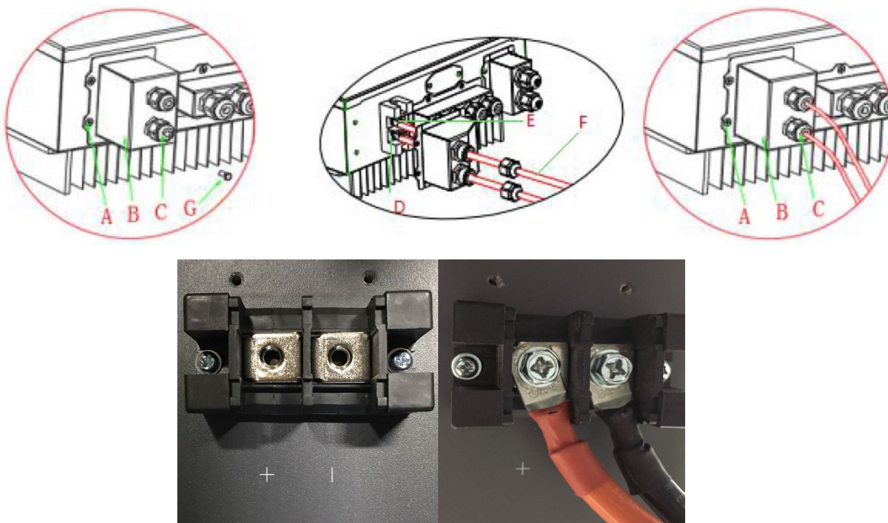
Figure 10 – Connexion d'alimentation de la batterie
