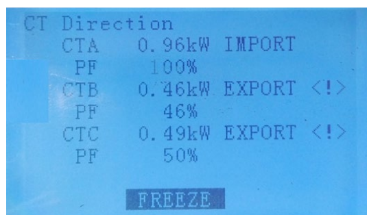
Figure 87 – Cas des sondes CTb et CTc installées sur des phases incorrectes
