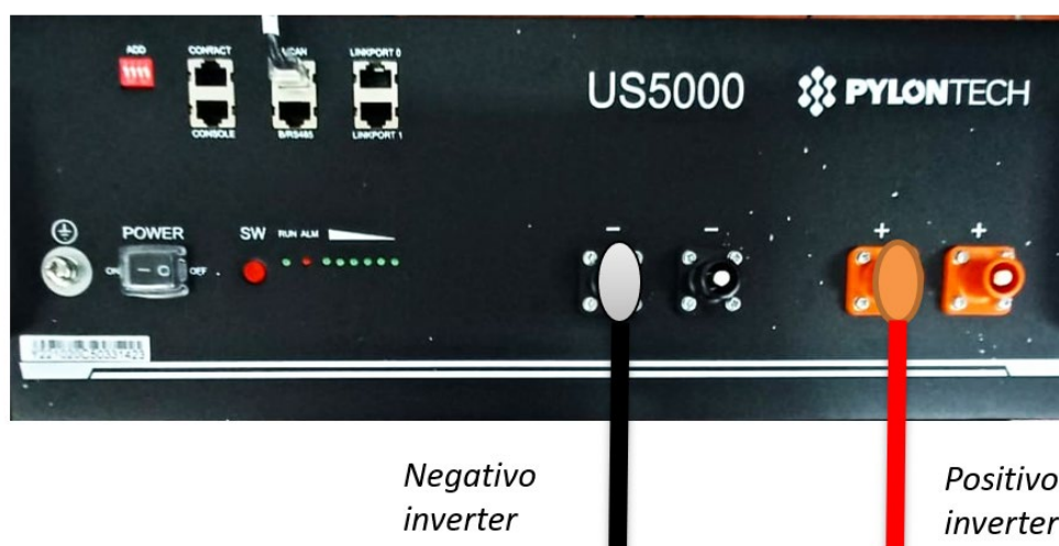
Figure 12- Connexion du câble d'alimentation de la batterie Pylontech à l'onduleur
