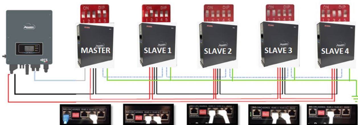
Figure 17 – Parallèle de cinq batteries WeCo 4k4
