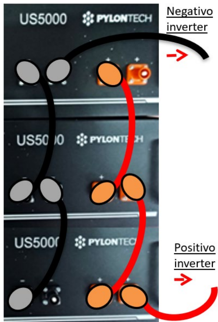
Figure 13 – Parallèle de trois batteries Pylontech
