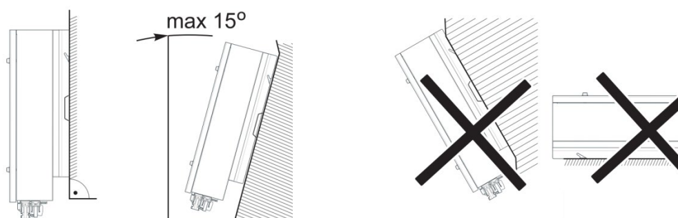
Figure 5 – Positionnement correct de l'onduleur 3000SP
