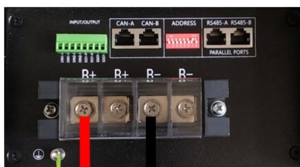
Figure 18 – Connexion de la batterie WeCo 4k4 LT
