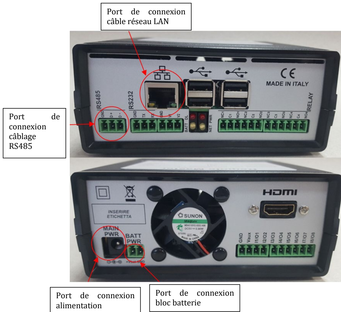
Figure152 : Vue arrière datalogger
