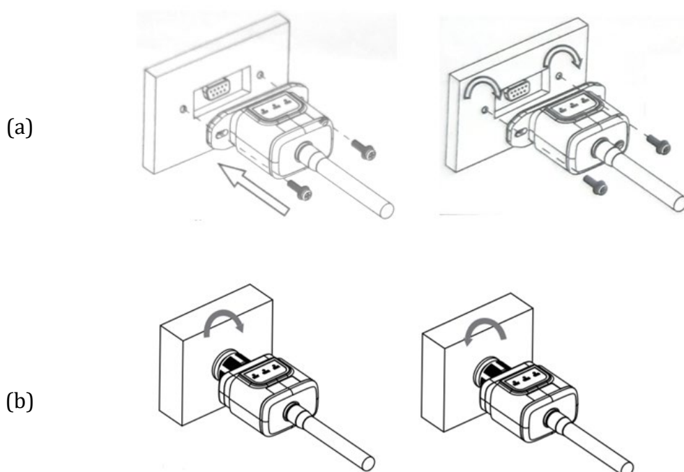
Figure 91 – Introduction et fixation de la carte Wi-Fi externe
