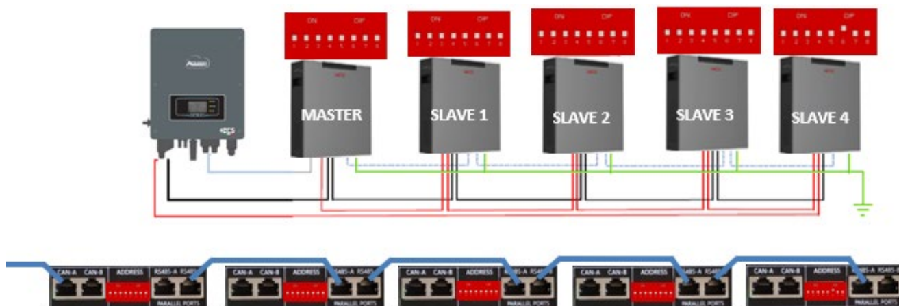
Figure 24 – Connexion en parallèle de cinq batteries WeCo 4k4-LT
