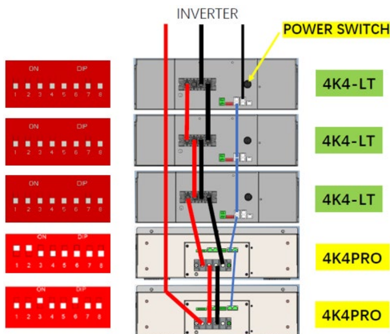
Figure 25 – Connexion batteries WeCo 4k4-LT et 4k4 PRO
