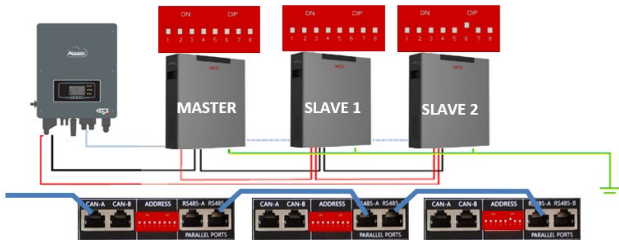
Figure 22 – Connexion en parallèle de trois batteries WeCo 4k4-LT
