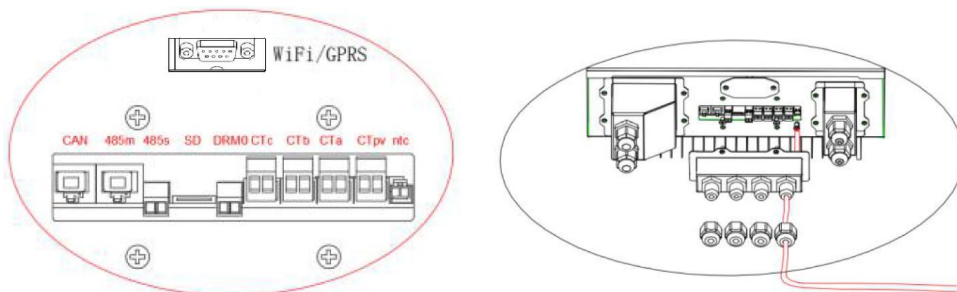
Figure 56 – Connexions des câbles CT pour les sondes de courant
