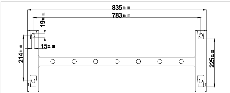
Figura -32 Dimensiones
