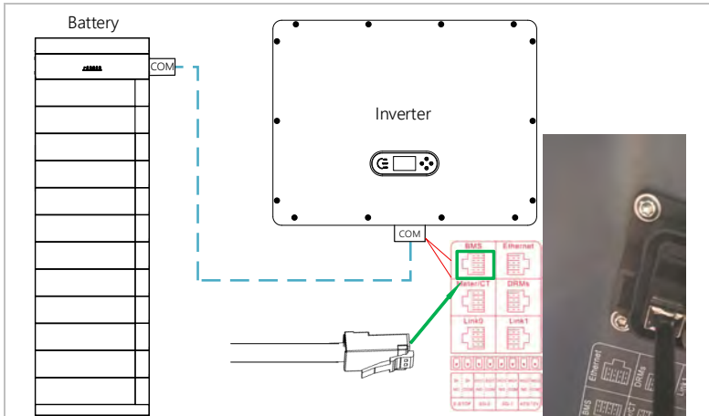
Figura 5-30 Conexión BMS
