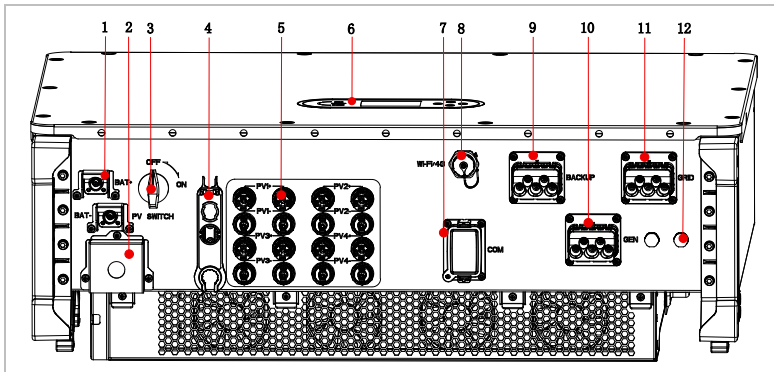
Figura -41 AZZURRO 3PH HYD 30000...60000 Descripción general del inversor ZSR
