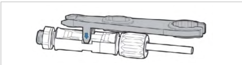
Figura5 -14 Conexión de PV(f)
