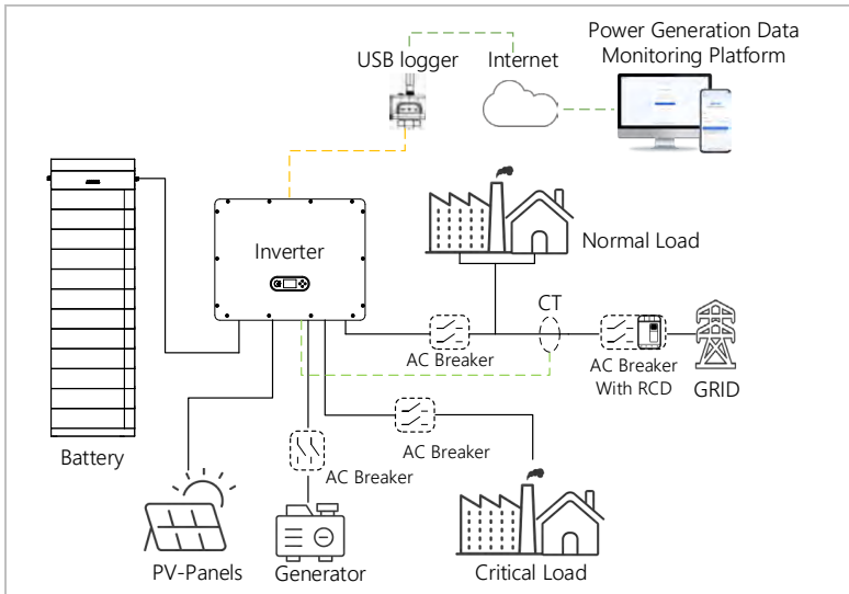
Figura -31 Diagrama del sistema del inversor AZZURRO 3PH HYD 30000...60000 ZSR
