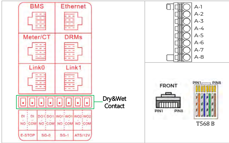
Figura5 -20 Interfaces COM
