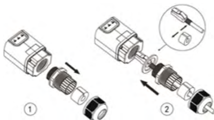
Figura 5-57 - Inserción del cable de red en el interior del dispositivo
