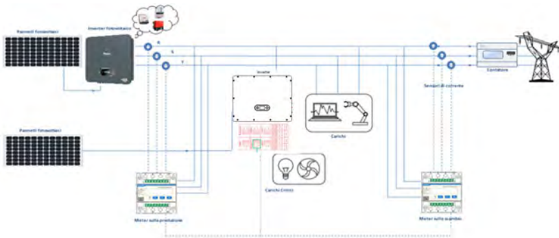
Figura 5-27a Conexión y medidor inteligente con CT en intercambio y producción (tomando como ejemplo el medidor inteligente CHINT)
