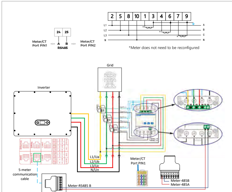
Figura 5-27 Conexión y medidor inteligente con CT (tomando como ejemplo el medidor inteligente CHINT)
