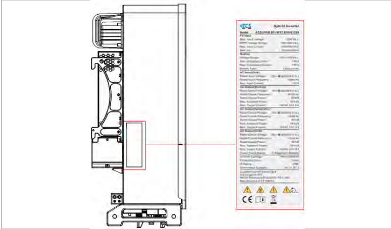
Figura -33 AZZURRO 3PH HYD 30000...60000 ZSR aspecto y etiqueta
