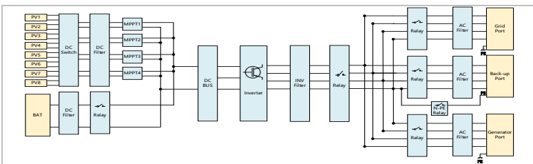
Figure -34 Schéma électrique
