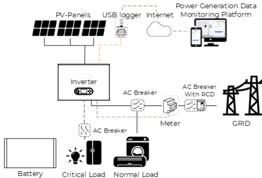
Figura 11 – Sistema senza batterie
