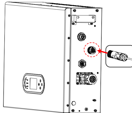
Figura 39 - Collegamento EPS
