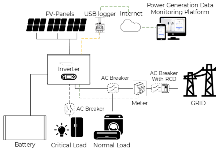
Figura 1 - Schema di un impianto su cui è installato un 3PH HYD5000-12000-ZP3 ibrido
