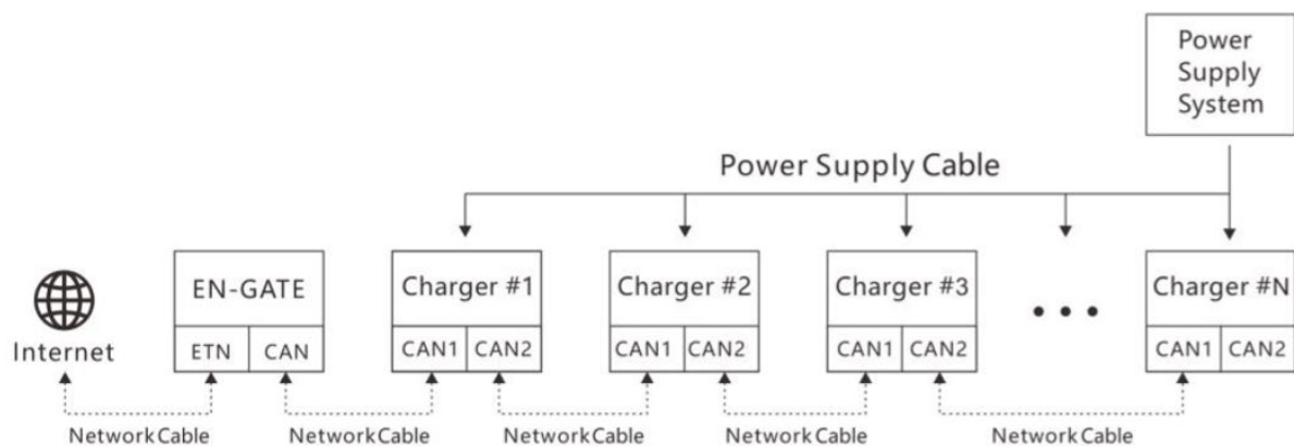
Figura 38 - Conexión entre ZVM-GATEWAY y cargadores
