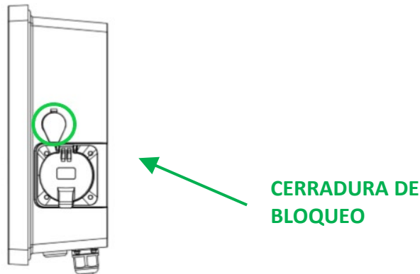
Figura 19 - Vista lateral del cargador
