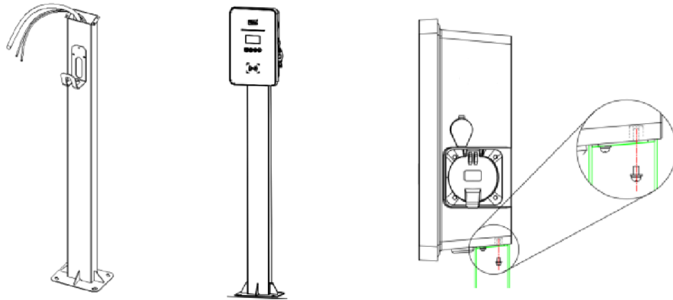
Рис. 16 -- Розташування опорного стовпа
