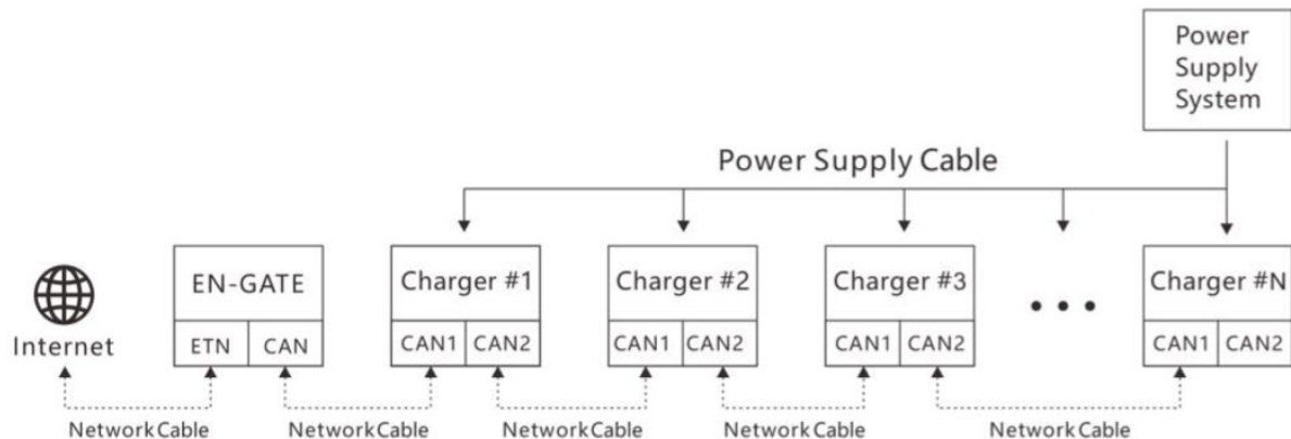
Рис. 37 - Зв'язок між ZVM-GATEWAY і зарядним пристроями
